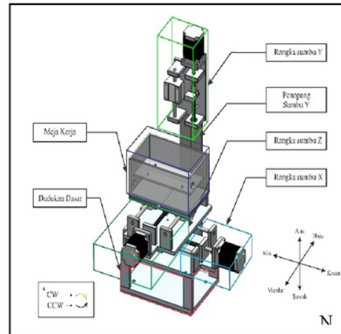
Gambar 1. Disain Mesin ECM dalam CAD
