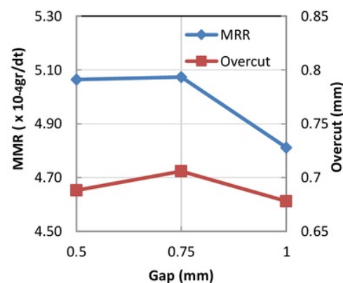
Gambar 6. Pengaruh gap terhadap MRR dan overcut ,
