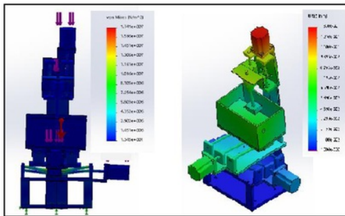
Gambar 5. Hasil simulasi (a) pembebanan dan (b) defleksinya
