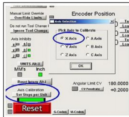
Gambar 3. Setting kalibrasi Mach 3 secara otomatis
