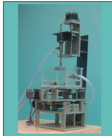
Gambar 2. Konstruksi sistem mekanikal Mesin ECM.
