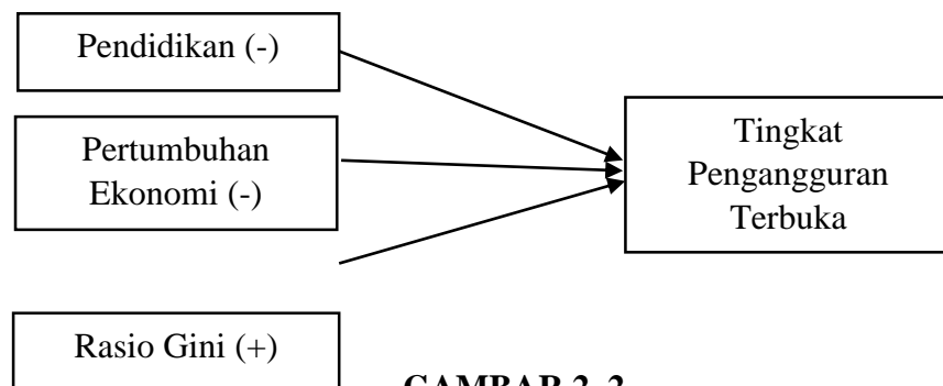
GAMBAR 2. 2 Kerangka Berfikir
