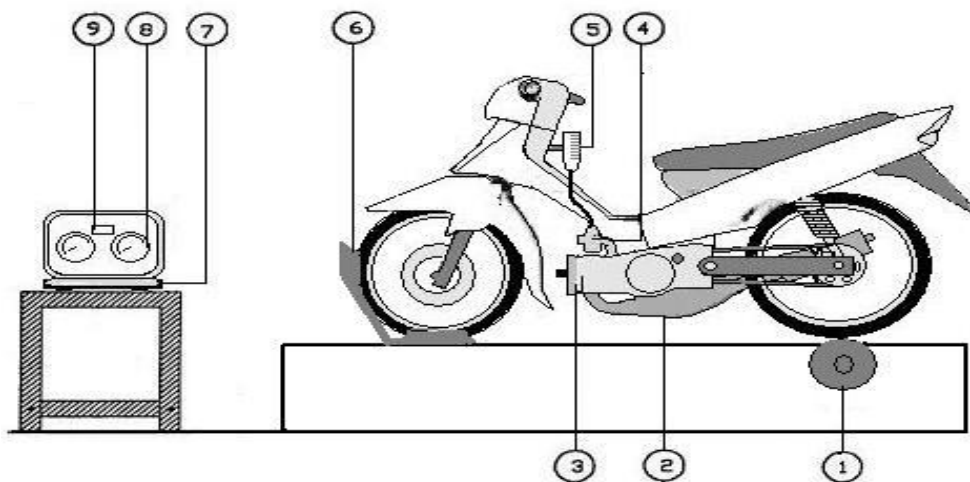
Gambar 3.12. Skema alat uji daya motor ( Singgih, 2013)
