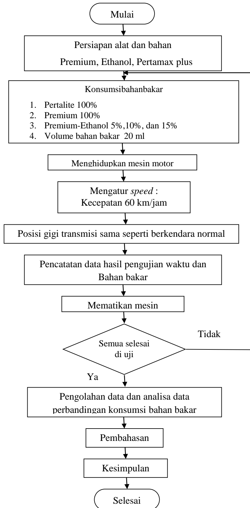
Gambar 3.10. Diagram Aliran Pengujian Konsumsi Bahan Bakar.
