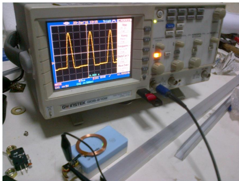
8. Pengukuran Output Transmitter Tanpa Beban
