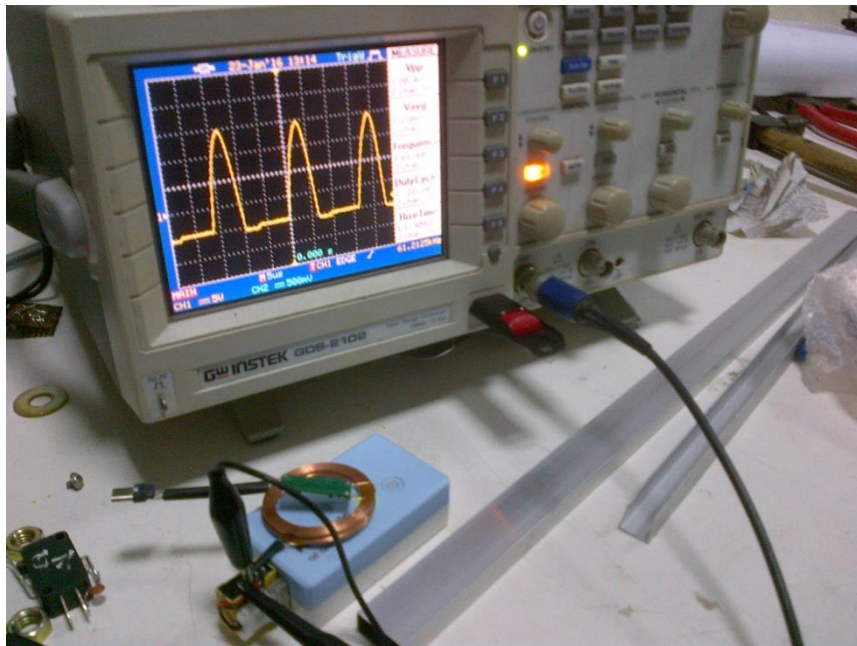
9. Pengukuran Output Transmitter dengan Receiver Tanpa Beban
