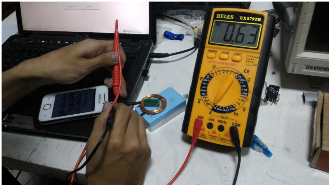
5. Pengukuran Input pada Telepon Genggam
