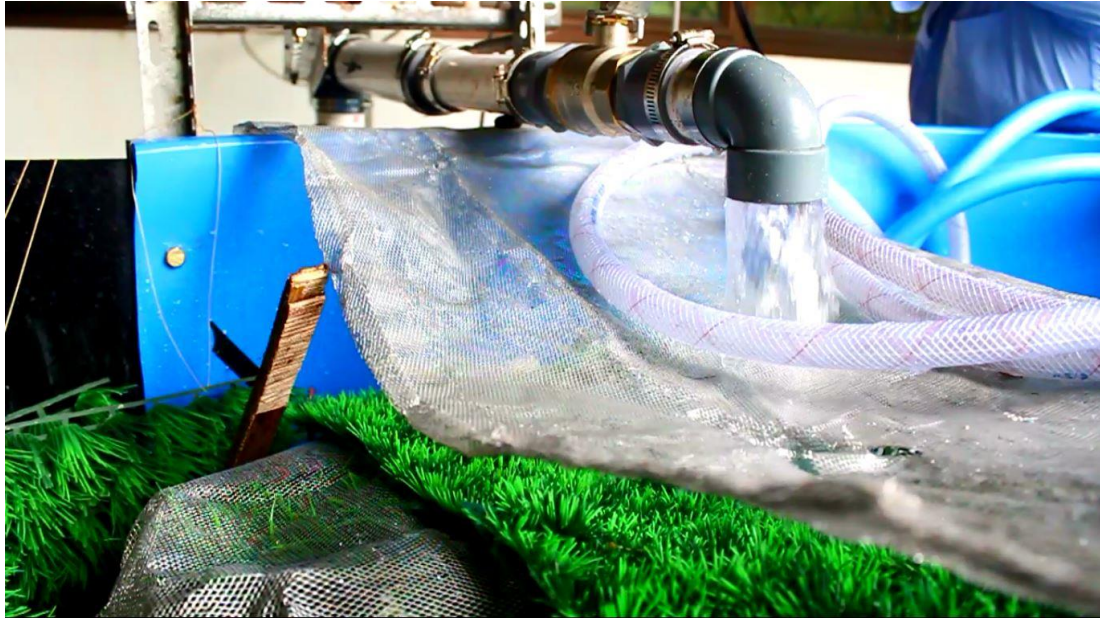
Peredam aliran
