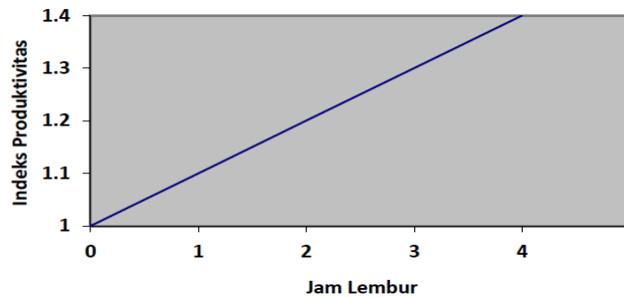
Gambar 3. 1 Grafik indikasi kenaikan produktivitas akibat penambahan jam kerja (Sumber: Soeharto, 1997)
