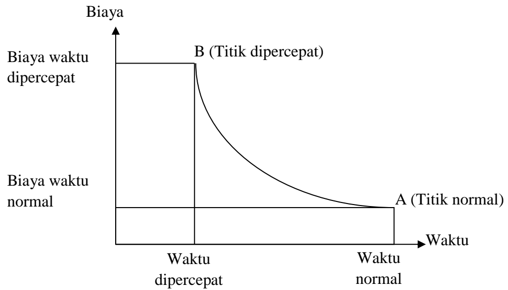
Gambar 3. 2 Hubungan waktu-biaya normal dan dipercepat untuk suatu kegiatan (Sumber: Soeharto, 1997)
