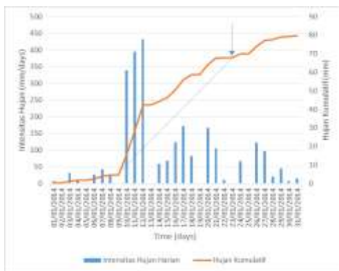
Gambar 1.3 Grafik intensitas hujan kumulatif di lokasi 3.
