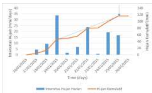
Gambar 1.71 Grafik intensitas hujan kumulatif di lokasi 71.
