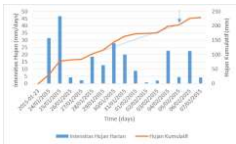
Gambar 1.41 Grafik intensitas hujan kumulatif di lokasi 41.
