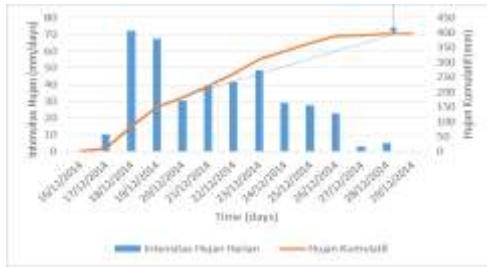
Gambar 1.85 Grafik intensitas hujan kumulatif di lokasi 85.
