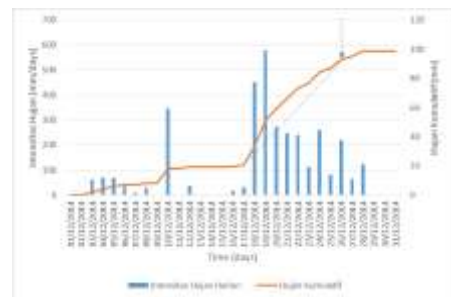
Gambar 1.42 Grafik intensitas hujan kumulatif di lokasi 42.
