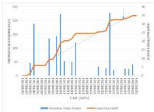
Gambar 1.77 Grafik intensitas hujan kumulatif di lokasi 77.
