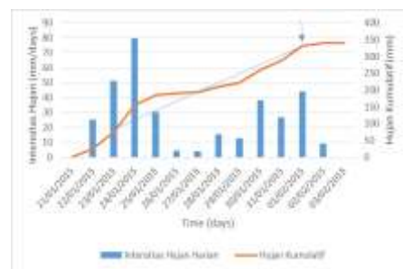
Gambar 1.52 Grafik intensitas hujan kumulatif di lokasi 52.
