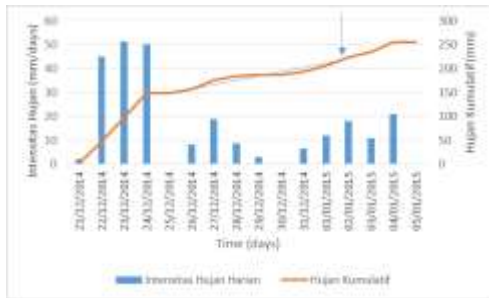
Gambar 1.79 Grafik intensitas hujan kumulatif di lokasi 79.
