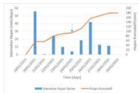
Gambar 1.76 Grafik intensitas hujan kumulatif di lokasi 76.
