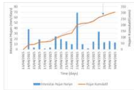
Gambar 1.8 Grafik intensitas hujan kumulatif di lokasi 8.
