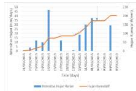
Gambar 1.48 Grafik intensitas hujan kumulatif di lokasi 48.
