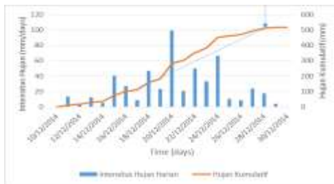
Gambar 1.89 Grafik intensitas hujan kumulatif di lokasi 89.
