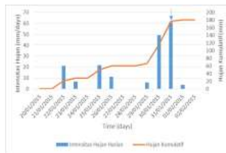
Gambar 1.58 Grafik intensitas hujan kumulatif di lokasi 58.
