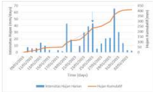
Gambar 1.73 Grafik intensitas hujan kumulatif di lokasi 73.
