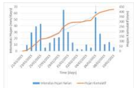
Gambar 1.34 Grafik intensitas hujan kumulatif di lokasi 34.
