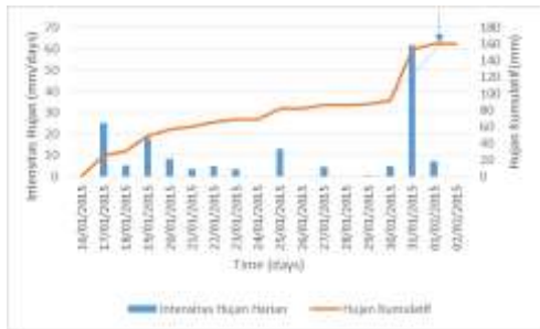
Gambar 1.49 Grafik intensitas hujan kumulatif di lokasi 49.
