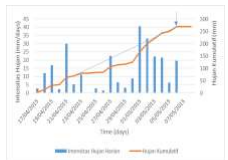
Gambar 1.6 Grafik intensitas hujan kumulatif di lokasi 6.
