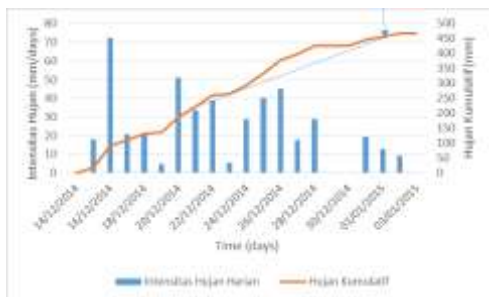
Gambar 1.83 Grafik intensitas hujan kumulatif di lokasi 83.
