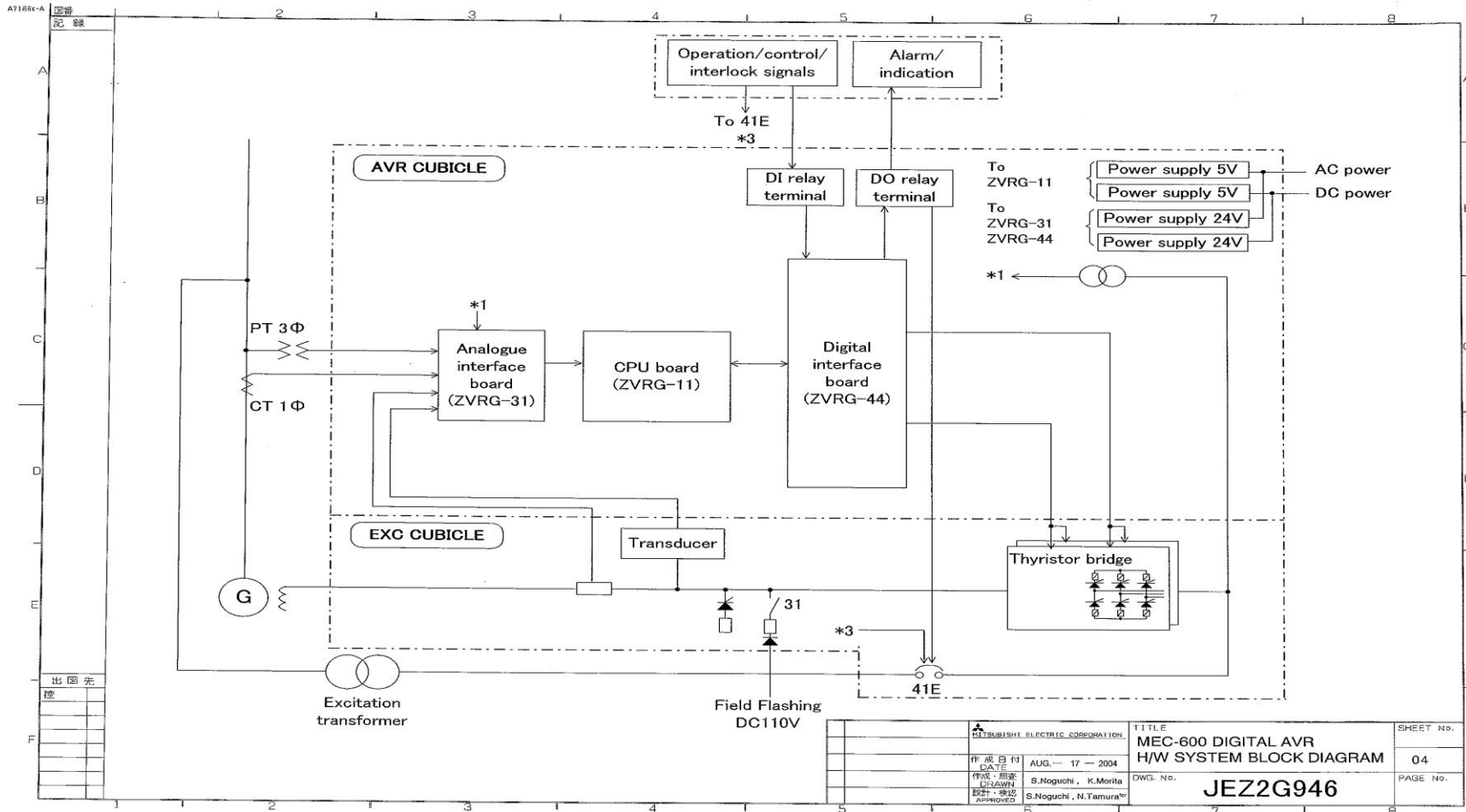
Lampiran 2 : Blok Diagram Sistem Eksitasi PLTA Musi
