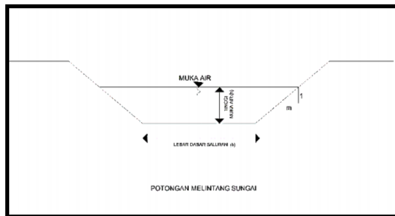
Gambar 3.3 Lebar saluran (potongan melintang)
