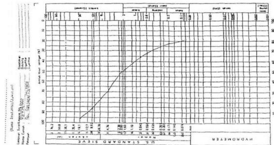
Gambar 3.4 Kurva distribusi ukuran butiran
