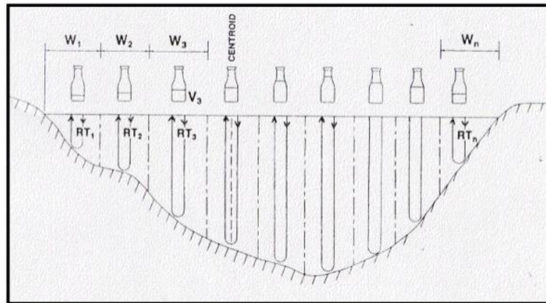
Gambar 3.7 Pengambilan sampel sedimen dengan cara EWI
