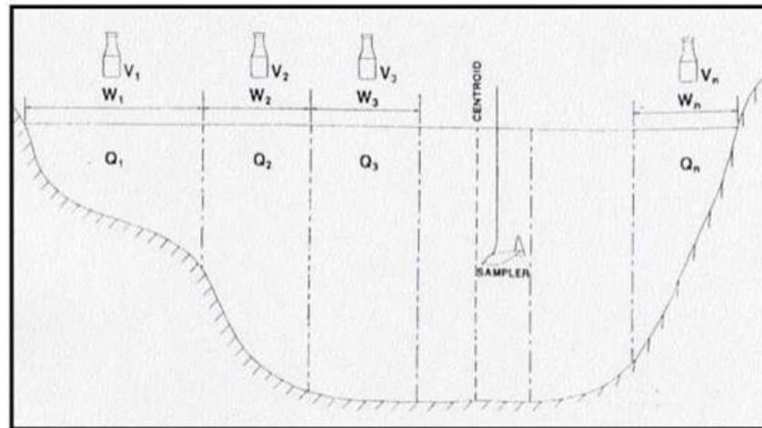
Gambar 3.6 Pengambilan sampel sedimen dengan cara EDI
