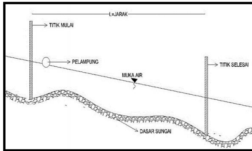
Gambar 3.1 Metode pengukuran kecepatan aliran dengan pelampung ( float ) (Sri Harto,2000)
