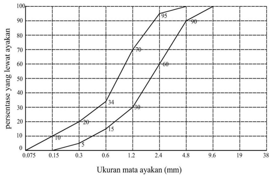
Gambar 3.5 Batas gradasi pasir pada daerah no.1 (SNI 03-2834-2000)
