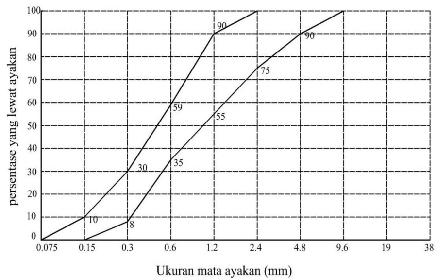
Gambar 3.6 Batas gradasi pasir pada daerah no.2 (SNI 03-2834-2000)
