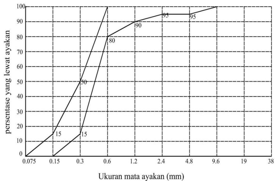
Gambar 3.8 Batas gradasi pasir pada daerah no.4 (SNI 03-2834-2000)
