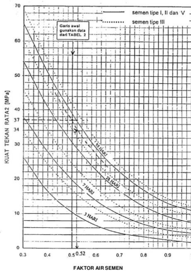
Gambar 3.4 Hubungan faktor air semen dan kuat tekan silinder beton (SNI 03-2834-2000)
