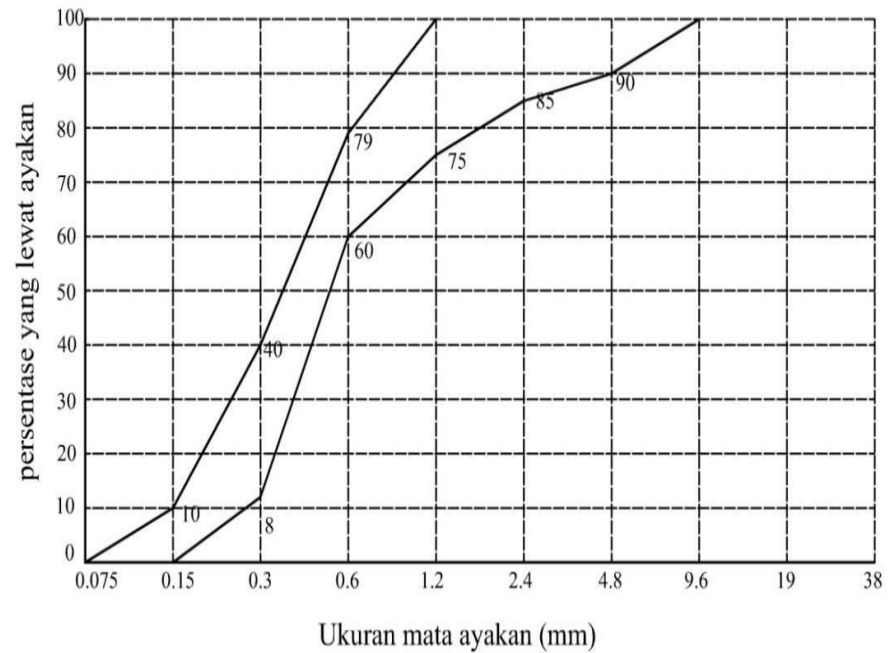
Gambar 3.7 Batas gradasi pasir pada daerah no.3 (SNI 03-2834-2000)
