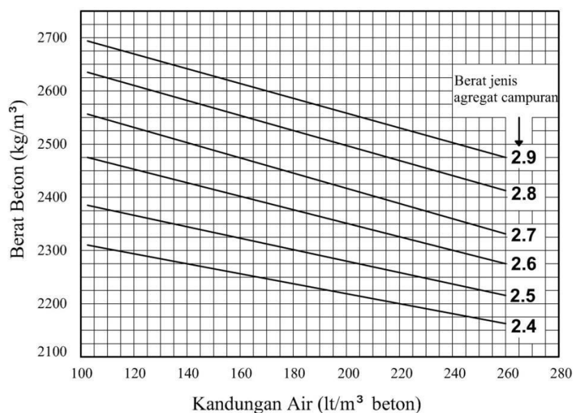
Gambar 3.10 Hubungan antara kandungan air, berat jenis agregat campuran dan berat beton (SNI 03-2834-2000)
