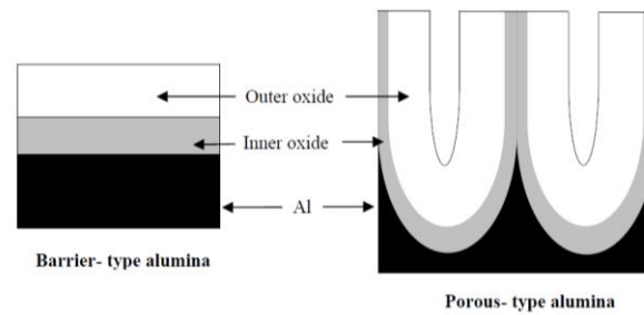
Gambar 2.6 Skema lapisan pori hasil anodisasi. (Rohman, 2012)
