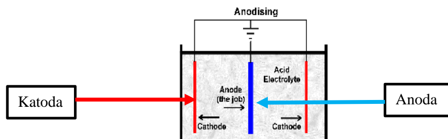
Gambar.2.1 Elektroda pada proses anodic oxidatio (Febriyanti, 2011).
