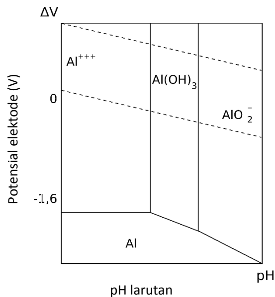
Gambar.2.8 Diagram porbeix alumunium (Diadopsi dari wikimedia.org)
