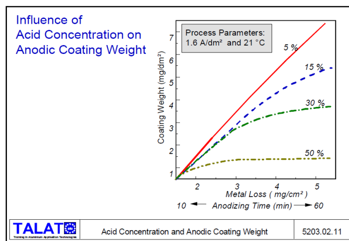
Gambar 2.4 Grafik waktu pencelupan anodizing terhadap berat lapisan oksida yang terbentuk dengan variasi konsentrasi elektrolit. (TALAT, 2009)
