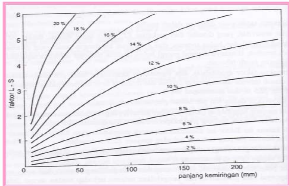
Gambar 3. 1Diagram untuk memperoleh nilai LS (suripin, dalam Hatas 2015)
