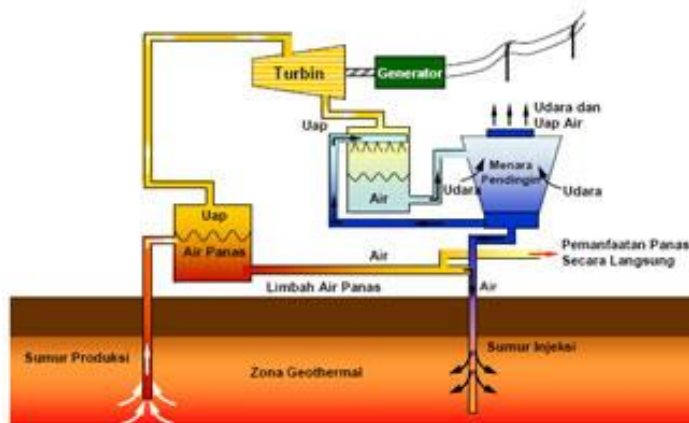
Gambar 2.6 Skema Sirkuit Uap dan Air Pada PLTP
