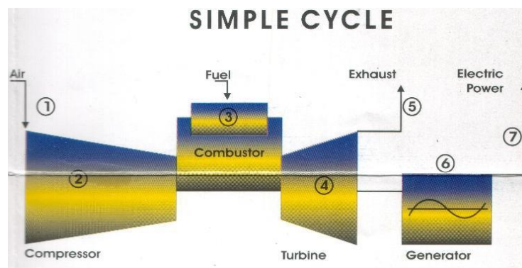
Gambar 2.2 Komponen Sistem Kerja PLTG
