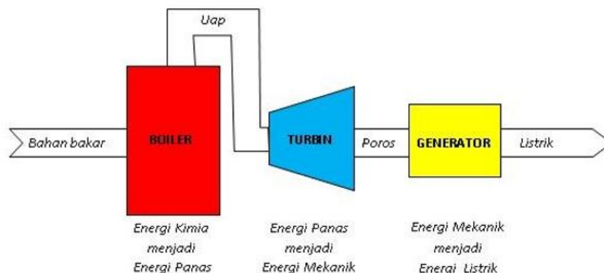
Gambar 2.7 Proses Konversi Energi pada PLTSa Sama Dengan PLTU
