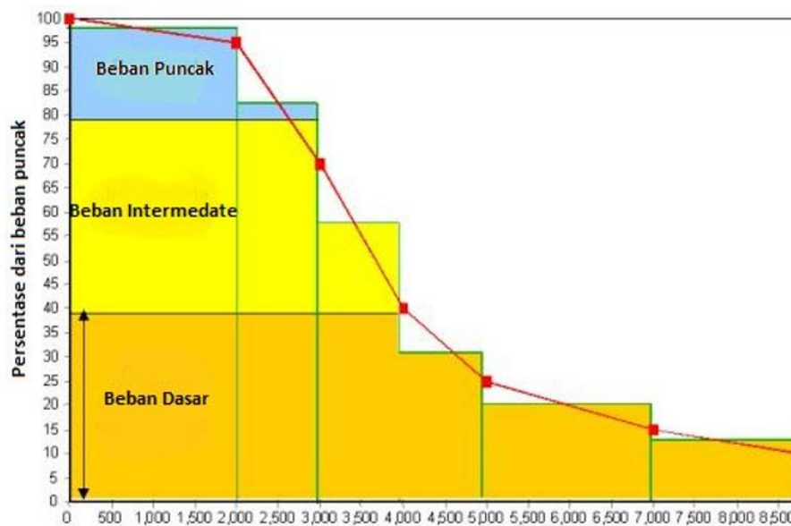
Gambar 2.10 Komulatif LDC
