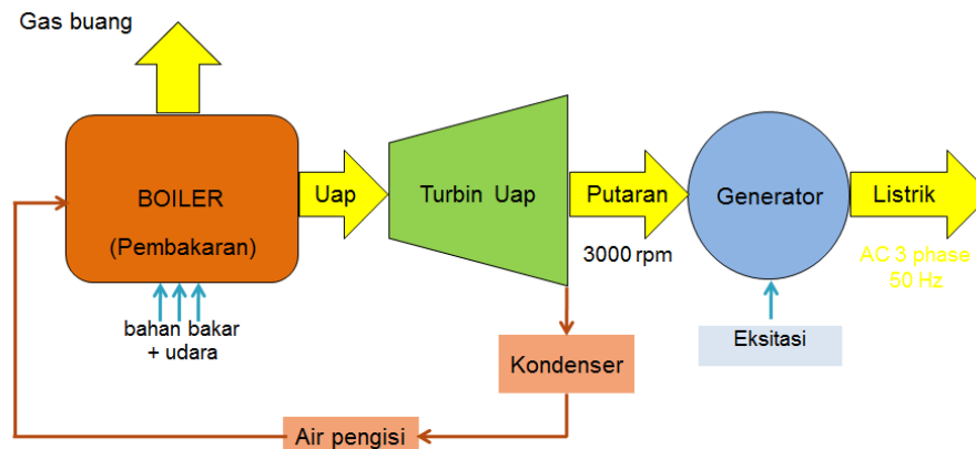
Gambar 2.1 Proses Konversi Energi PLTU
