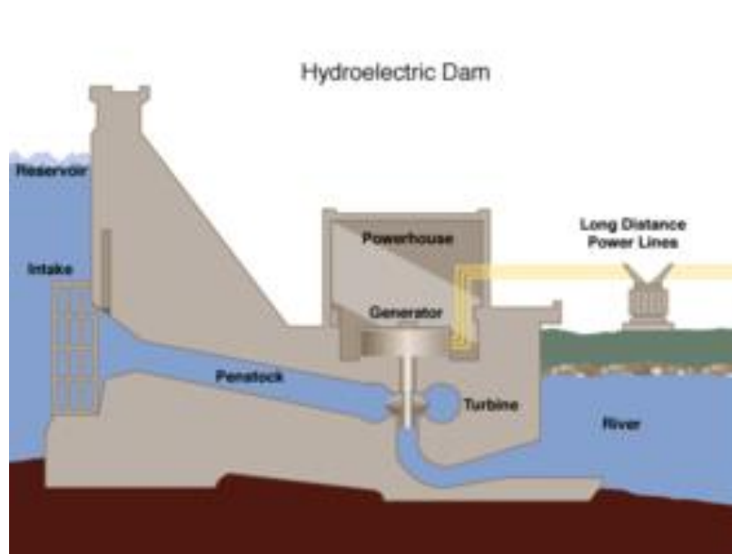
Gambar 2.5 Proses Konversi Energi pada PLTA
