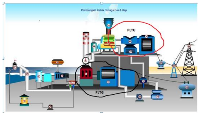
Gambar 2.3 Prinsip Kerja PLTGU
