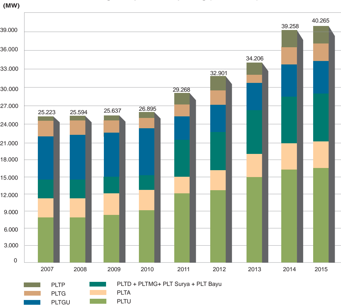
Grafik 7. Perkembangan Kapasitas Terpasang (2007 - 2015)
