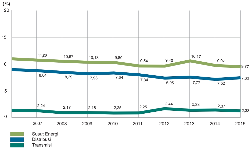
Grafik 6. Perkembangan Susut Energi (2007 - 2015)
