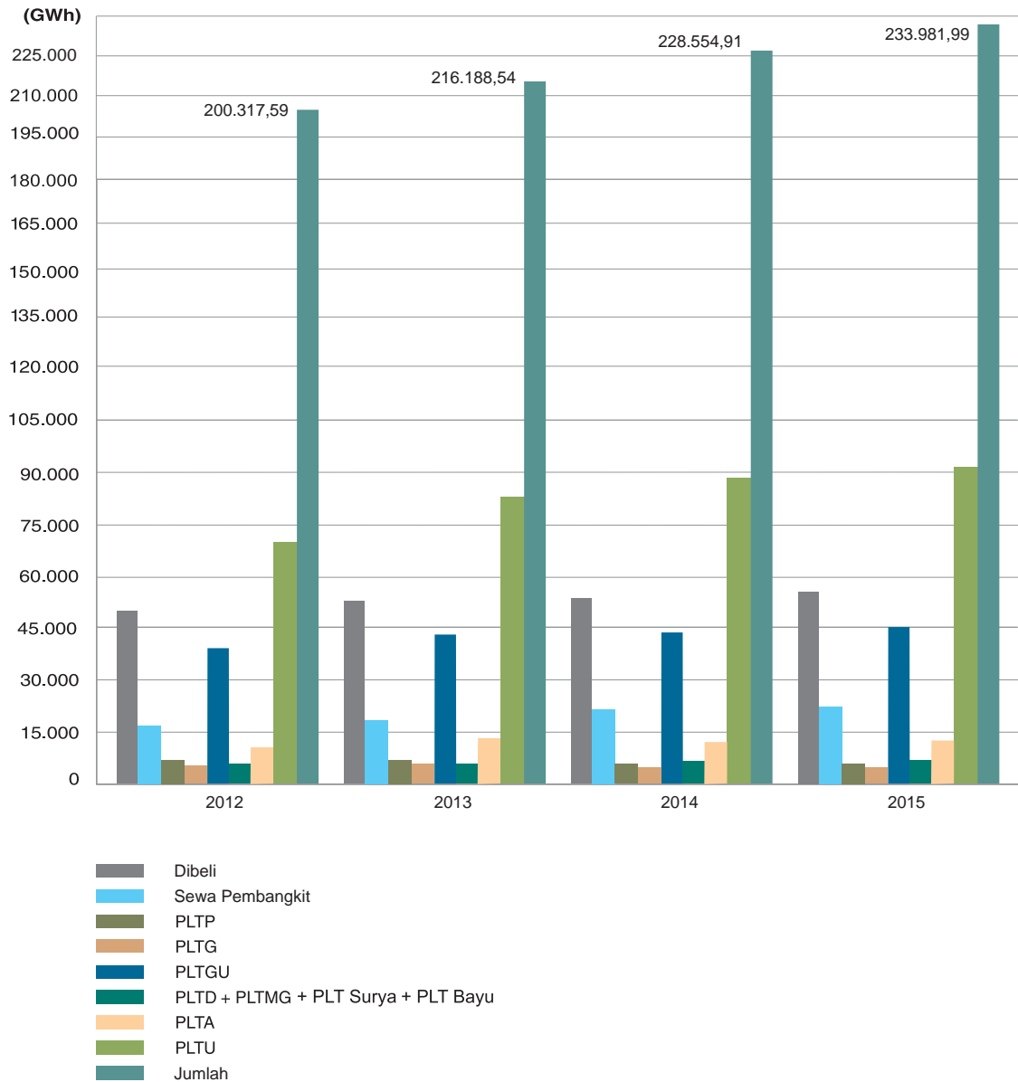
Grafik 8. Perkembangan Energi yang Diproduksi (2012 - 2015)
