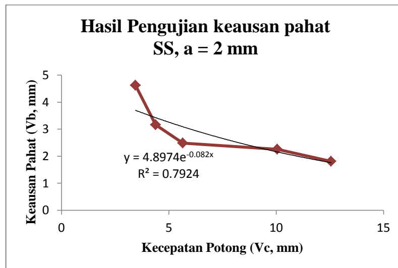
Gambar 4.16 Grafik perbandingan Vc dan Vb pada SS, a = 2.
