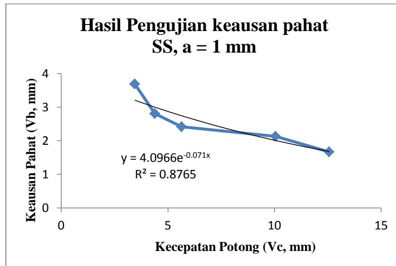
Gambar 4.15 Grafik perbandingan Vc dan Vb pada SS, a = 1
