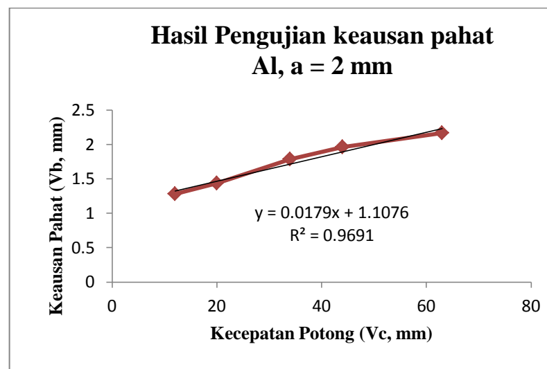
Gambar 4.14 Grafik perbandingan Vc dan Vb pada Al, a = 2
