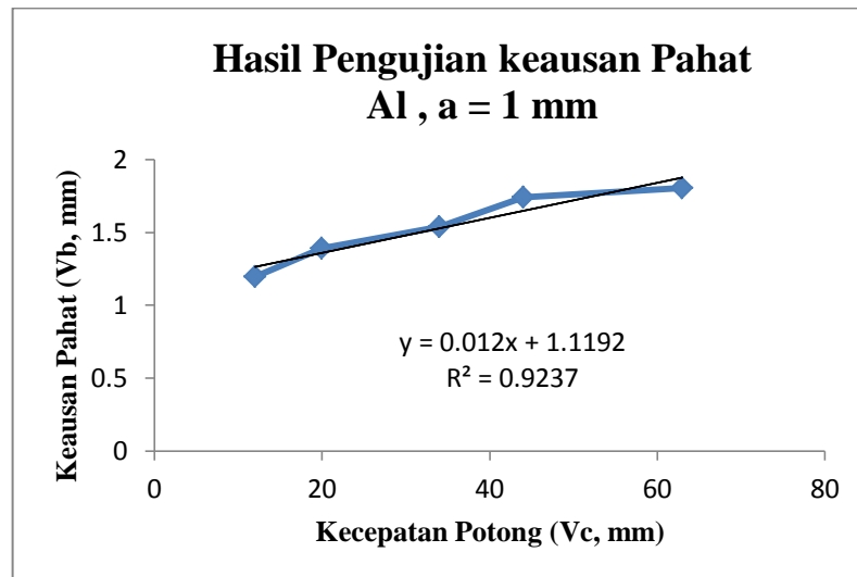
Gambar 4.13 Grafik perbandingan Vc da Vb pada Al, a = 1
