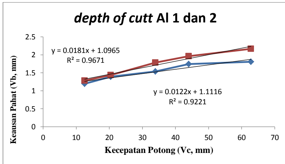
Gambar 4.17 Grafik Aluminium depth of cutt 1 dan 2.
