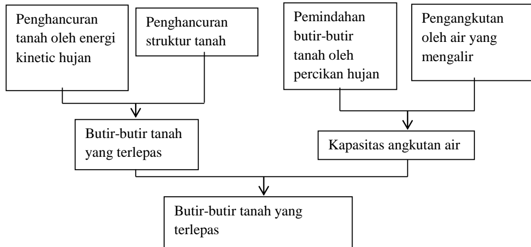
Gambar 2.2 Bagan alir model proses erosi oleh air (Suripin, 2004,dalam Hatas)
