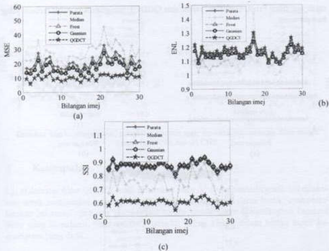
Gambar 2 Perbandingan hasil parameter statistik dalam mengurangiderau bintik (a) MSE, (b) ENL dan (c) SSI
