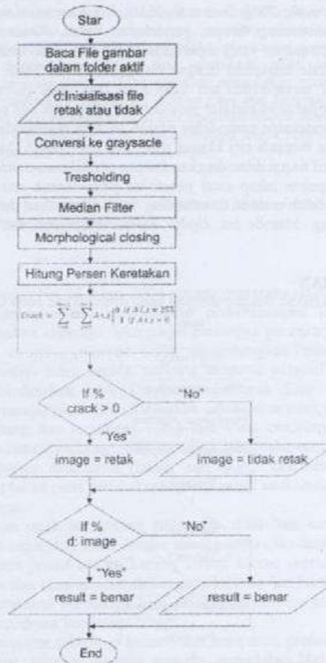
Gambar 2 Blok diagram perancangan algoritma
