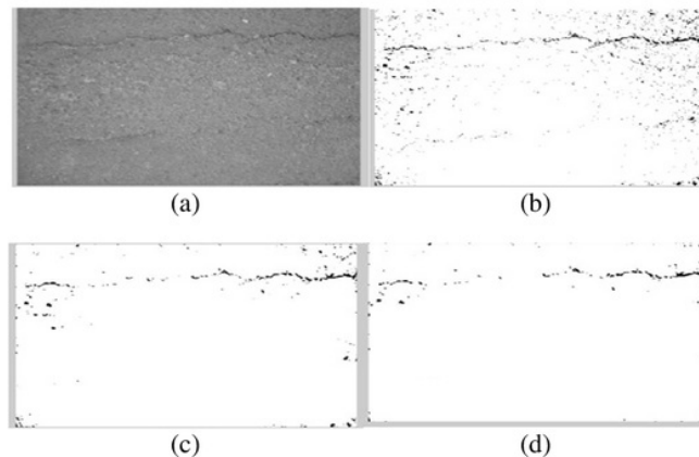
Gambar 3. Contoh citra hasil (a) konversi citra warna ke grayscale (b) thresholding (c) median filter dan (d) morphological closing
