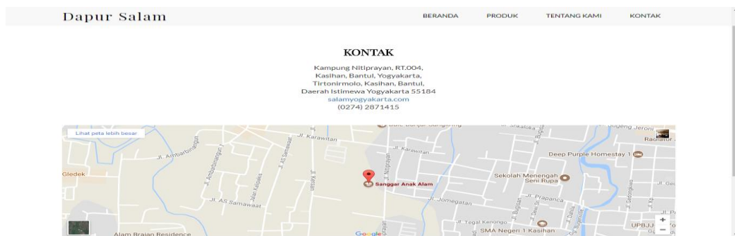
Gambar 4.16 Halaman Kontak
