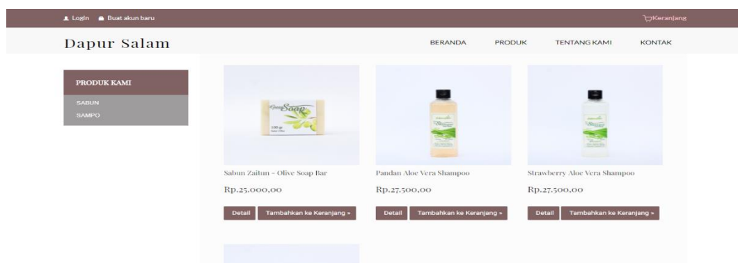
Gambar 4.12 Halaman Produk
