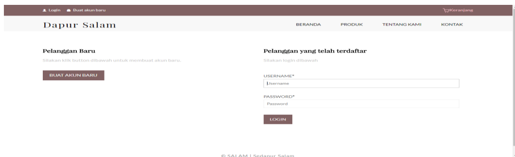
Gambar 4.18 Halaman Login
