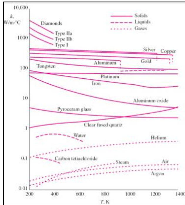
Gambar 2.19 Variasi konduktivitas termal berbagai jenis benda padat, cair dan gas pada berbagai temperatur (Cengel, 2011)
