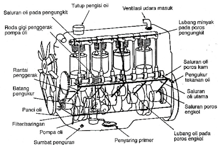
Gambar 2.11 Sistem pelumasan basah (Daryanto, 2004)
