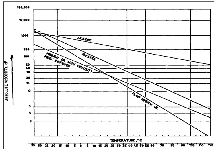
Gambar 2.18 Indeks viskositas dengan temperatur (Shigley, 2004)
