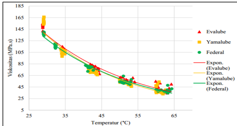
Gambar 2.1 Perbandingan 3 jenis oli terhadap nilai viskositas dan suhu (Inang, 2017)
