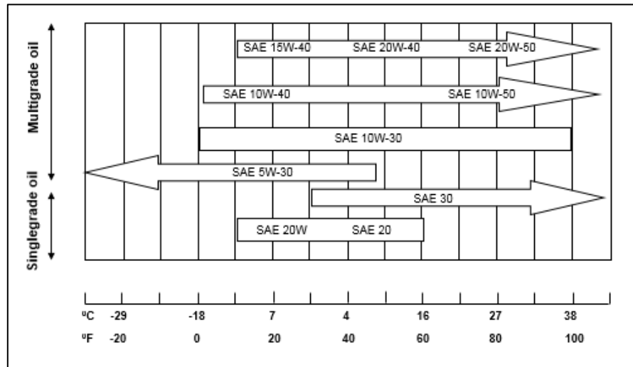
Gambar 2.6 Rekomendasi penggunaan oli motor (Subaru, 2016)
