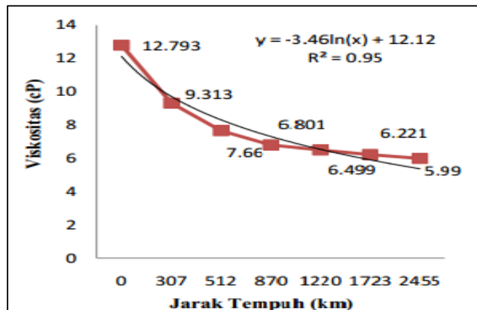
Gambar 2.3 Hubungan jarak tempuh dengan nilai viskositas pelumas pada sepeda motor (Wayan, 2015)
