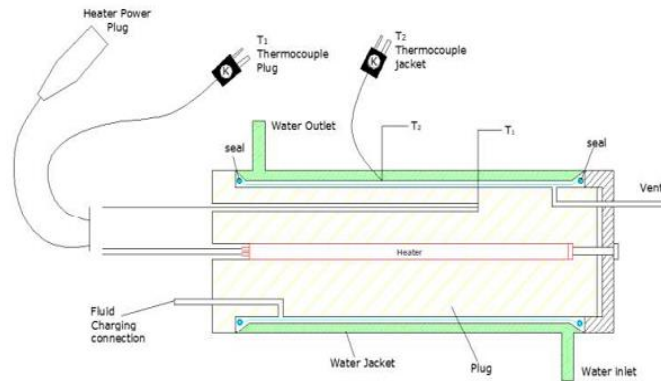
Gambar 2.20 Skema alat konduktivitas termal
