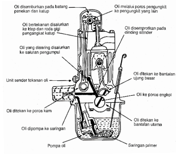
Gambar 2.13 Sistem pelumasan (Daryanto, 2004)
