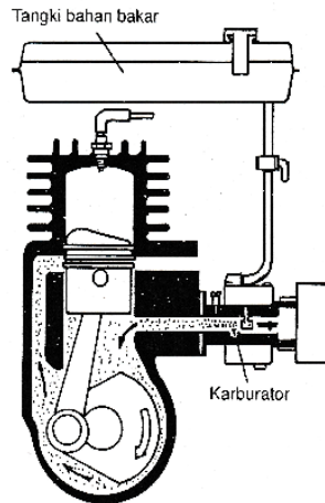
Gambar 2.9 Pelumasan campur bahan bakar (Daryanto, 2004)
