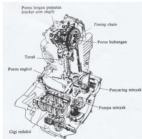
Gambar 2.12 Sistem pelumasan motor 4-langkah (Daryanto, 2004)
