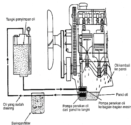
Gambar 2.10 Sistem pelumasan tipe kering (Daryanto, 2004)
