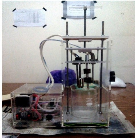
Gambar 3.3. Alat Pemanas dan Pengaduk
