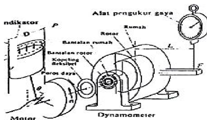
Gambar 2.13. Skema alat uji dinamometer (Purnomo, 2013)
