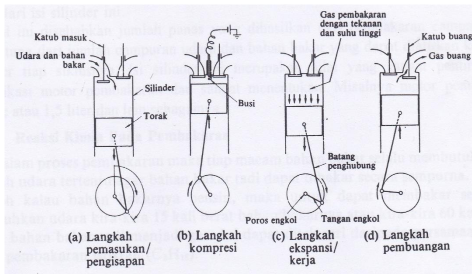
Gambar 2.12. Cara kerja motor 4-langkah (Daryanto, 2004)
