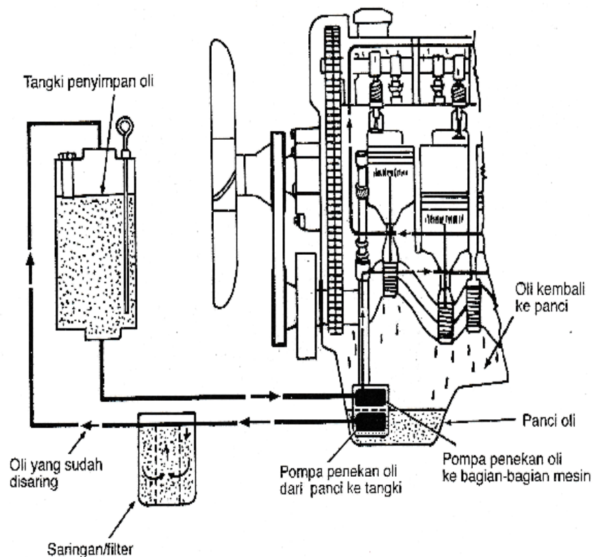
Gambar 2.8. Sistem pelumasan tipe kering (Daryanto, 2004)
