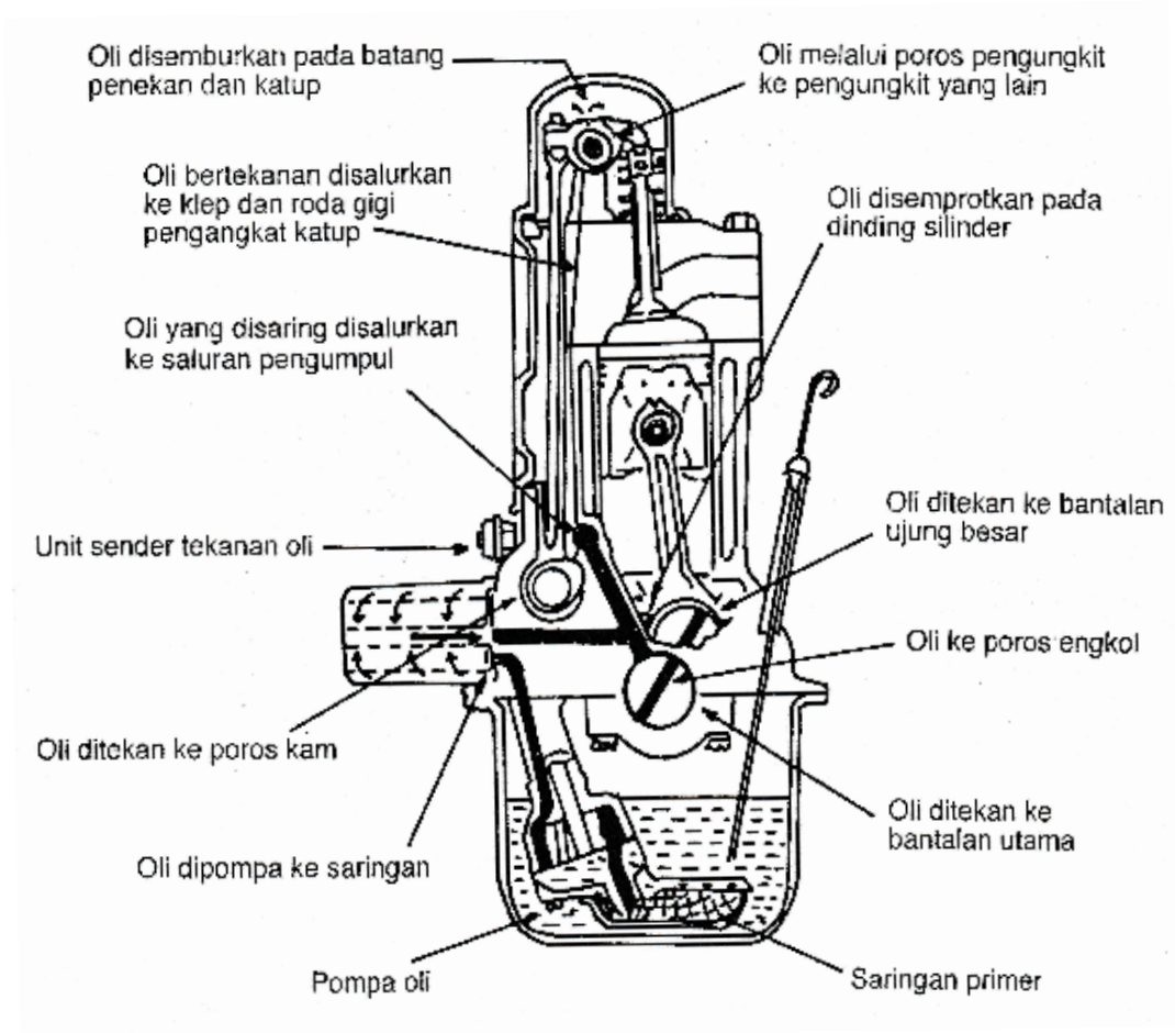
Gambar 2.11. Sistem pelumasan (Daryanto, 2004)
