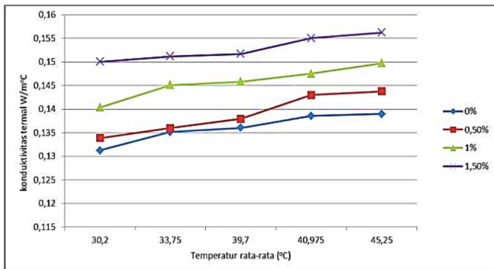
Gambar 2.3. Grafik hubungan antara temperatur dan fraksi volume terhadap konduktivitas termal (Irawansyah dan Kamal, 2012)
