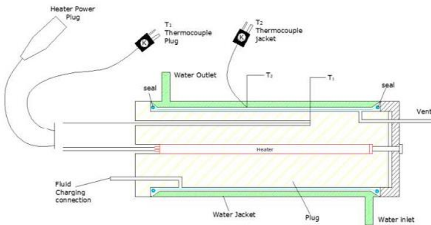
Gambar 2.6. Skema alat konduktivitas termal
