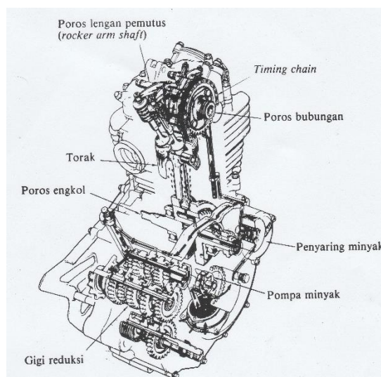
Gambar 2.10. Sistem pelumasan motor 4-langkah (Dayanto, 2004)
