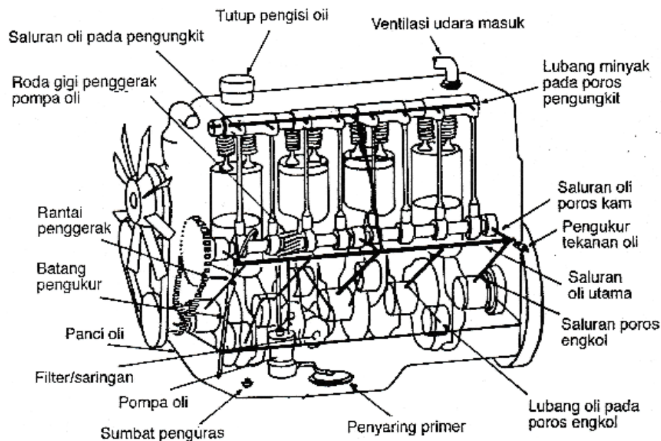
Gambar 2.9. Sistem pelumasan basah (Daryanto, 2004)
