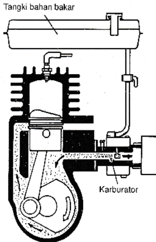
Gambar 2.7. Pelumasan campur bahan bakar (Daryanto, 2004)
