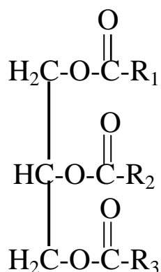
Gambar 2.5. Struktur Trigelisarida
