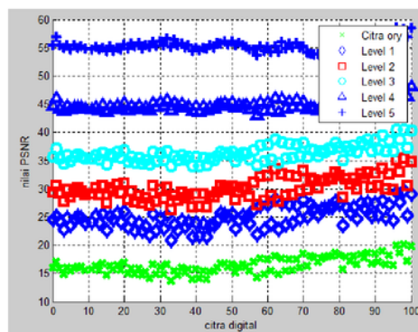
Gbr. 14 Parameter PSNR untuk Pyramida Gaussian
