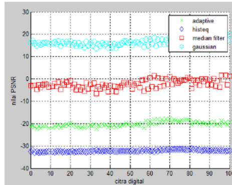
Gbr. 13 Parameter PSNR untuk CLAHE, HE, Median Filter dan Gaussian Filter
