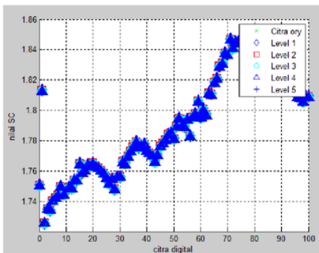
Gbr. 12 Parameter SC untuk Pyramida Gaussian
