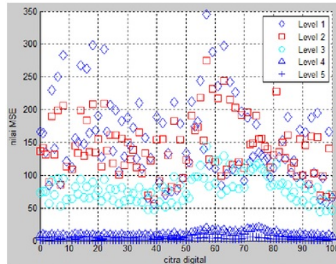
Gbr. 10 Parameter MSE untuk Pyramida Gaussian
