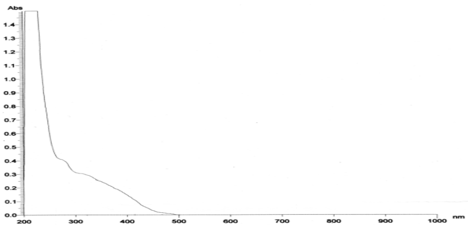
Gambar 5. Spektrum serapan isolat flavonoid dengan \text{AlCl}_3 .
