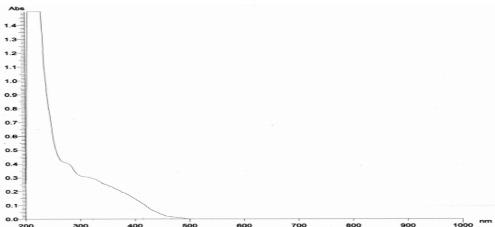
Gambar 6. Spektrum serapan isolat flavonoid dengan \text{AlCl}_3/\text{HCl} .
