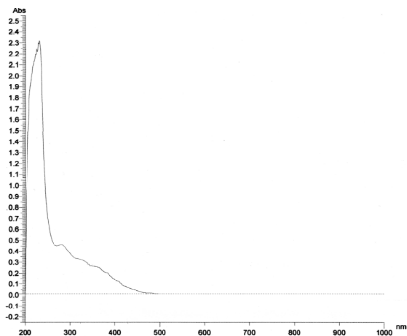
Gambar 4. Spektrum serapan isolat flavonoid dengan NaOAc/ H_3BO_3 .
