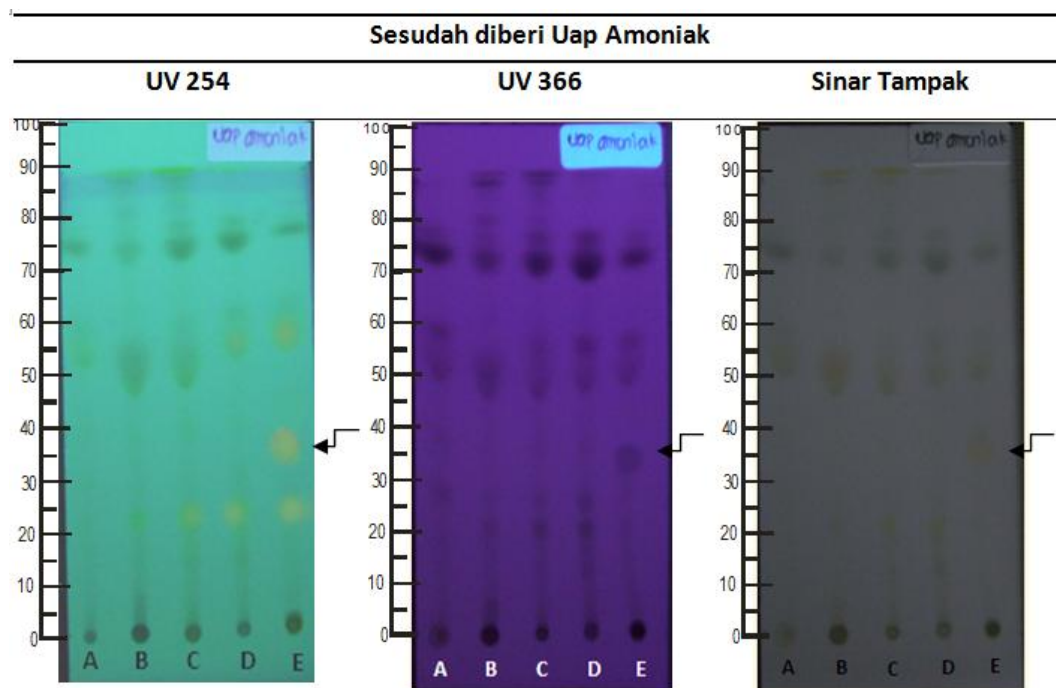
Gambar 1. Profil KLT sesudah diberi uap amonia. A=ekstrak daun Coccoloba uvifera (Anggur laut) sebagai pembanding, B=ekstrak daun Rheum officinale (Kelembak) sebagai pembanding, C=ekstrak daun Rumex acetosa (Rumex) sebagai pembanding, D=ekstrak daun Polygonum barbatum (Salah nyowo) sebagai pembanding, dan E=ekstrak daun Muehlenbeckia platyclada (Jakang) sebagai senyawa yang diidentifikasi.
