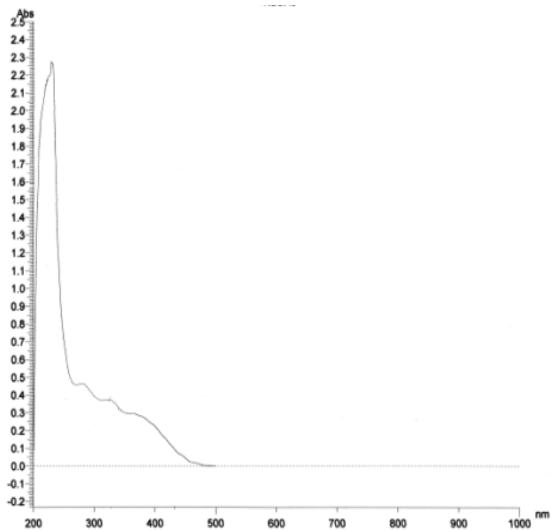
Gambar 3. Spektrum serapan isolat flavonoid dengan NaOAc.
