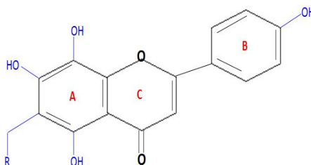
Gambar 7. Struktur parsial senyawa penanda daun jakang.
