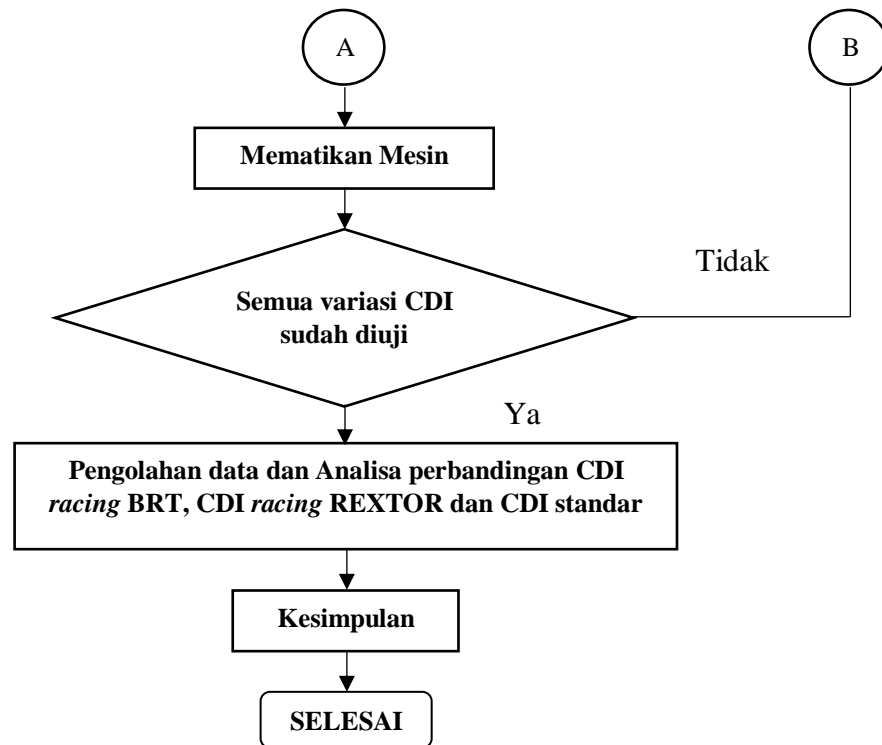
Gambar 3.20 Flow Chart pengujian Konsumsi Bahan Bakar (Lanjutan)
