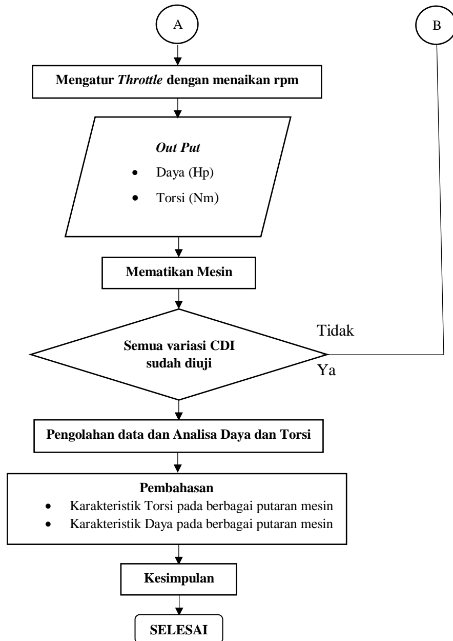
Gambar 3.19 Flow Chart pengujian Daya dan Torsi (Lanjutan)
