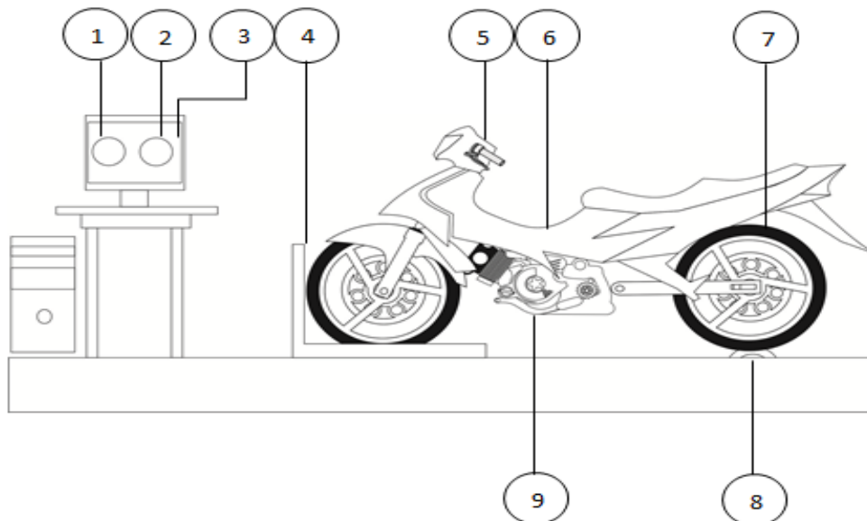
Gambar 3.21 Skema alat uji daya dan torsi motor
