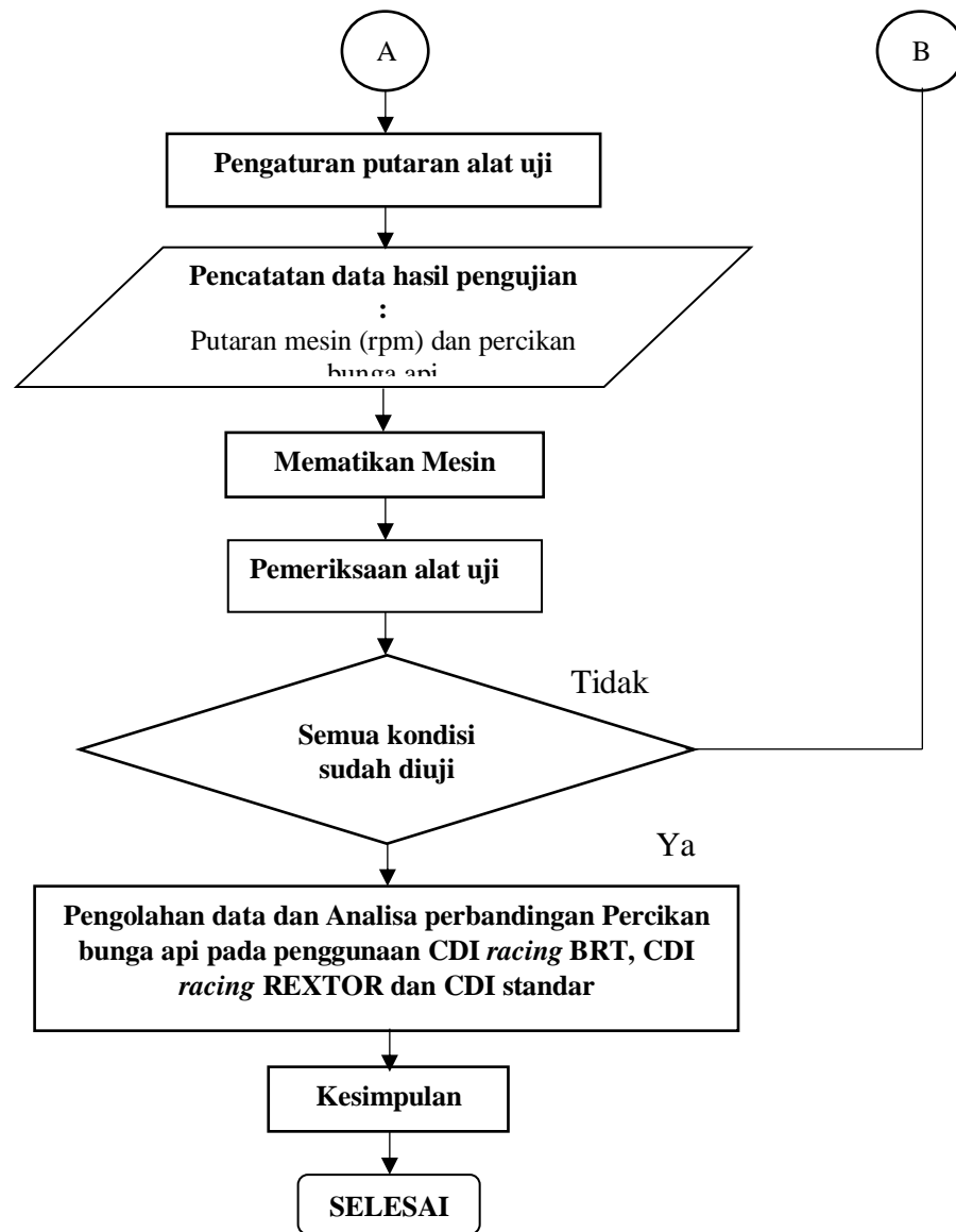
Gambar 3.18 Flow Chart pengujian Percikan Bunga Api Busi (Lanjutan)
