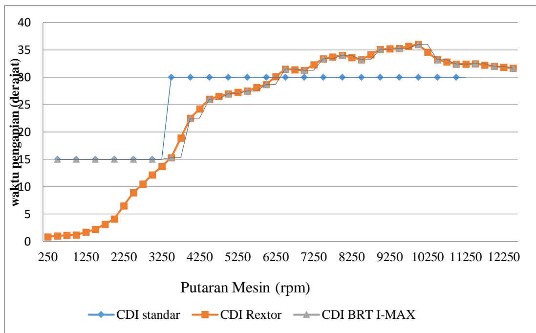
Gambar 3.4 Grafik Perbandingan waktu pengapian (Derajat) pada CDI standar, CDI racing Rextor da CDI racing BRT I-MAX
