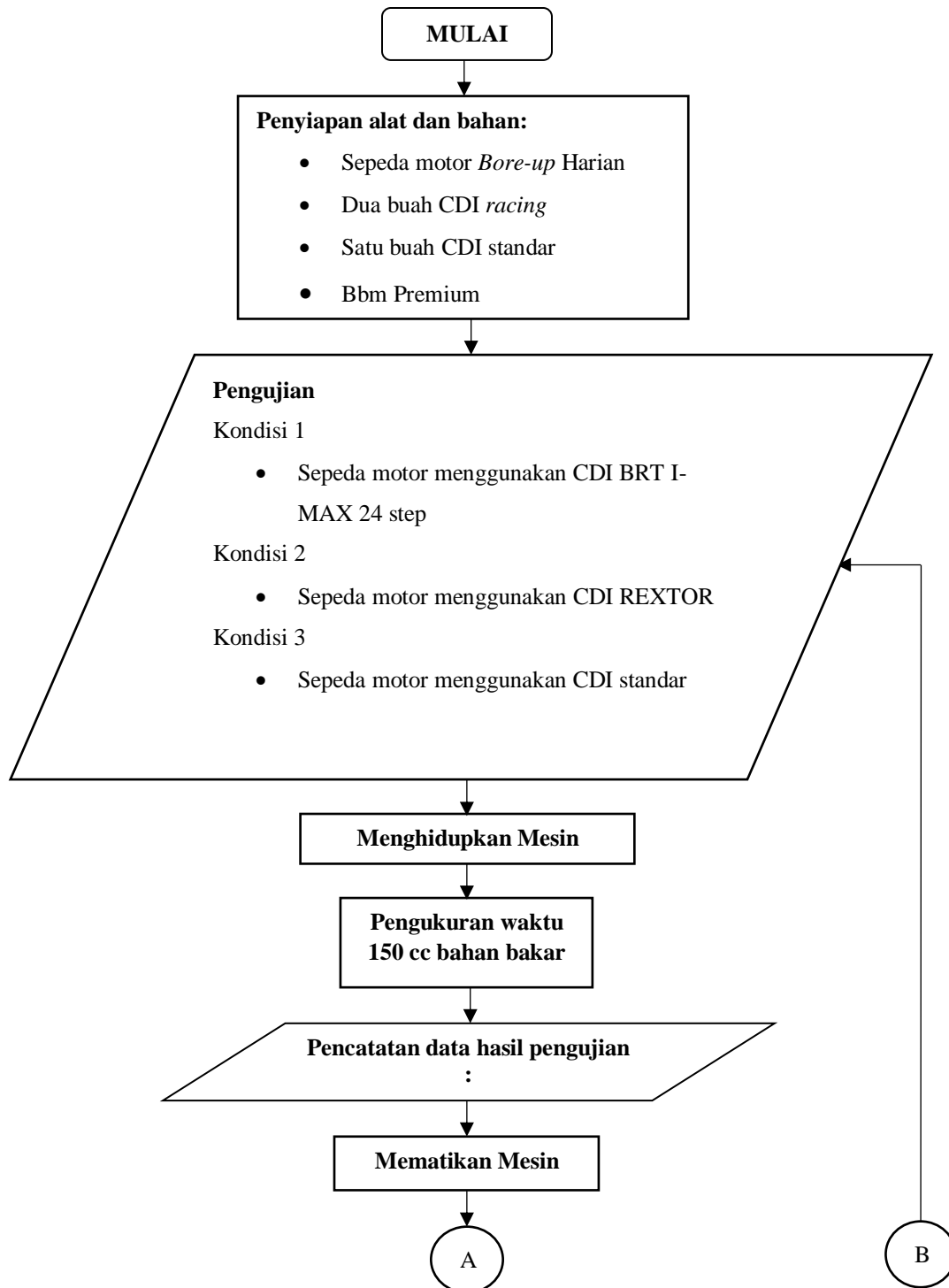
Gambar 3.20 Flow Chart pengujian Bahan Bakar
