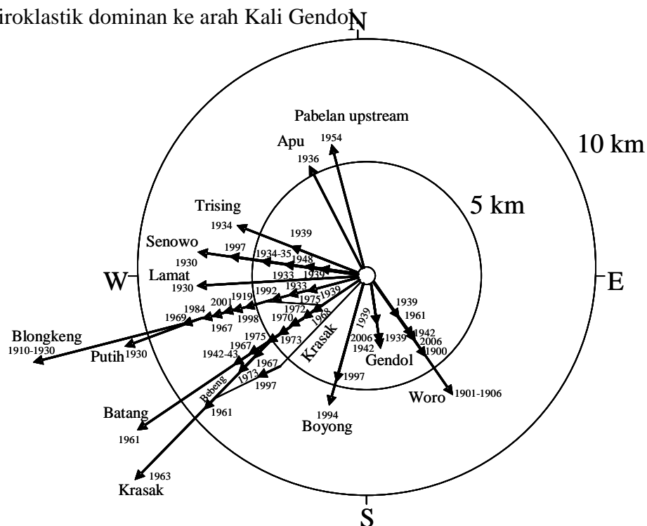
Gambar 2. Diagram arah kejadian aliran piroklastik (dimodifikasi dari DGWR 2001)
