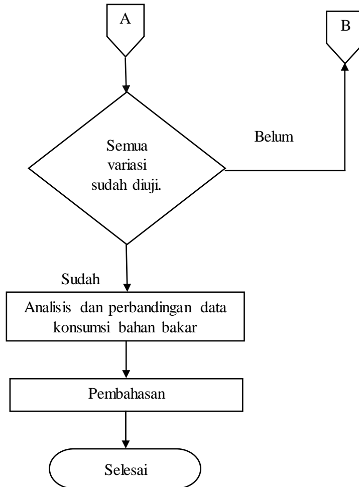
Gambar 3.22 Diagram alir pengujian konsumsi bahan bakar (lanjutan)
