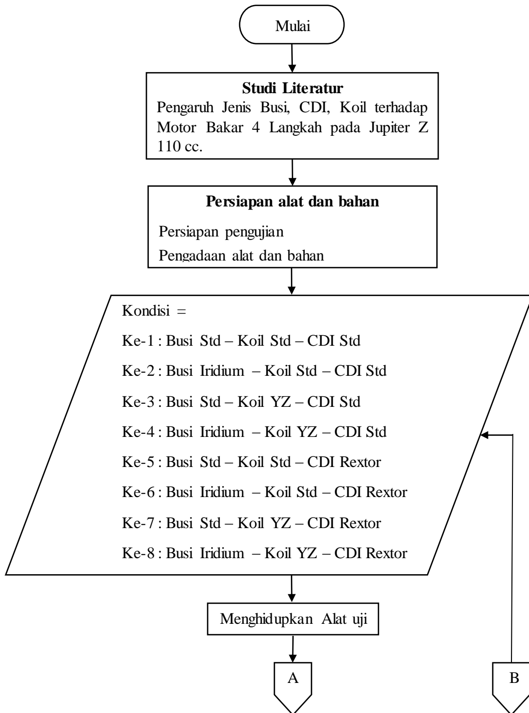
Gambar 3.3 Diagram alir pengujian percikan bunga api busi
