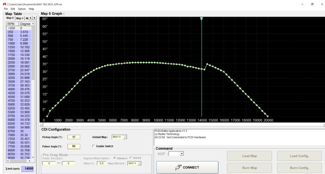
Gambar 3.20 Grafik mapping CDI programmable
