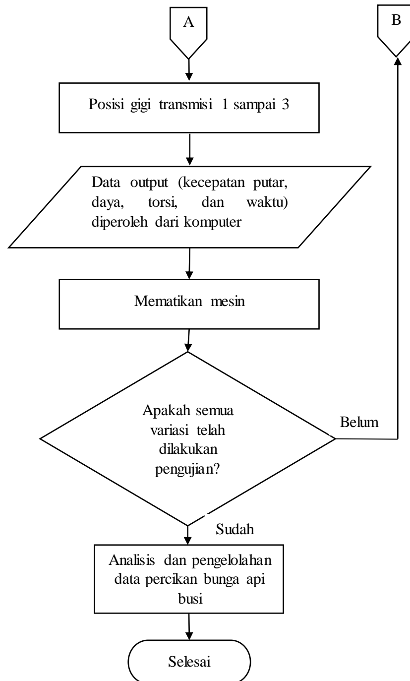
Gambar 3.7 Diagram alir pengujian daya dan torsi (lanjutan)
