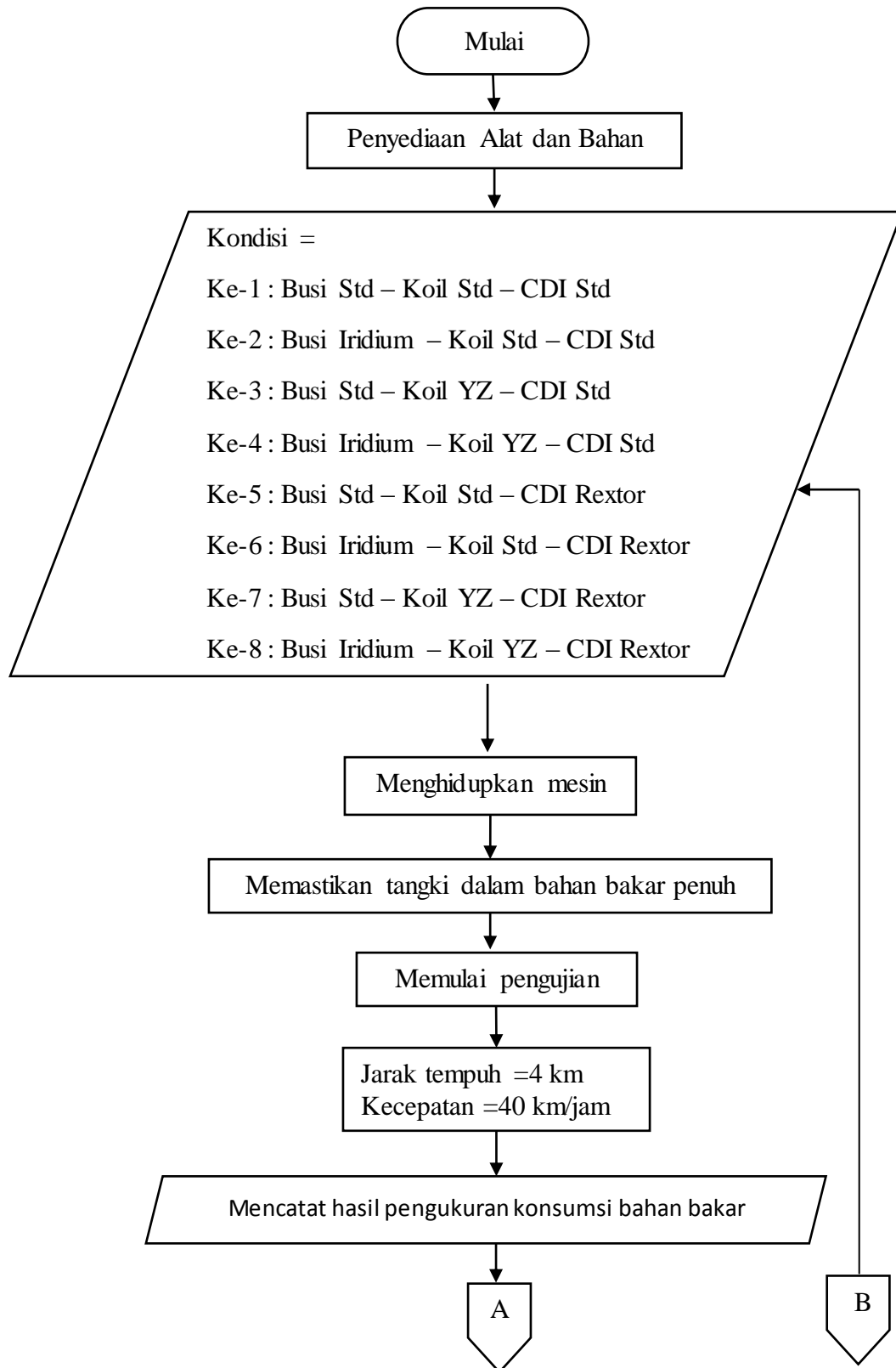
Gambar 3.21 Diagram alir pengujian konsumsi bahan bakar
