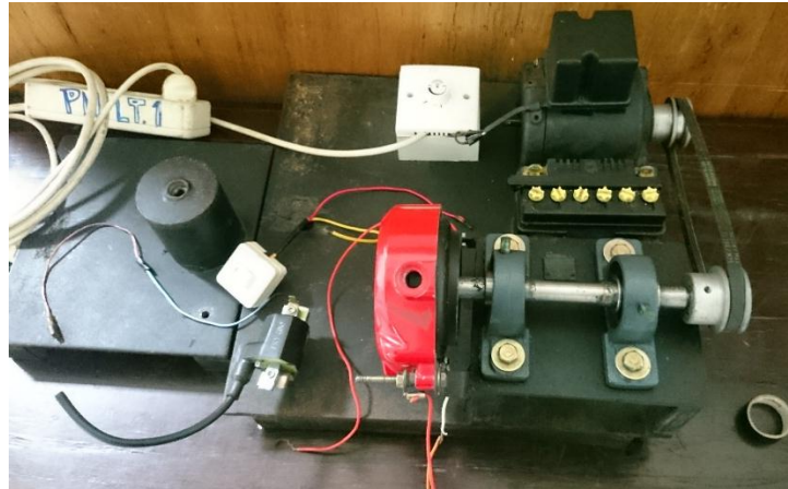
Gambar 3.5 Alat uji percikan bunga api
