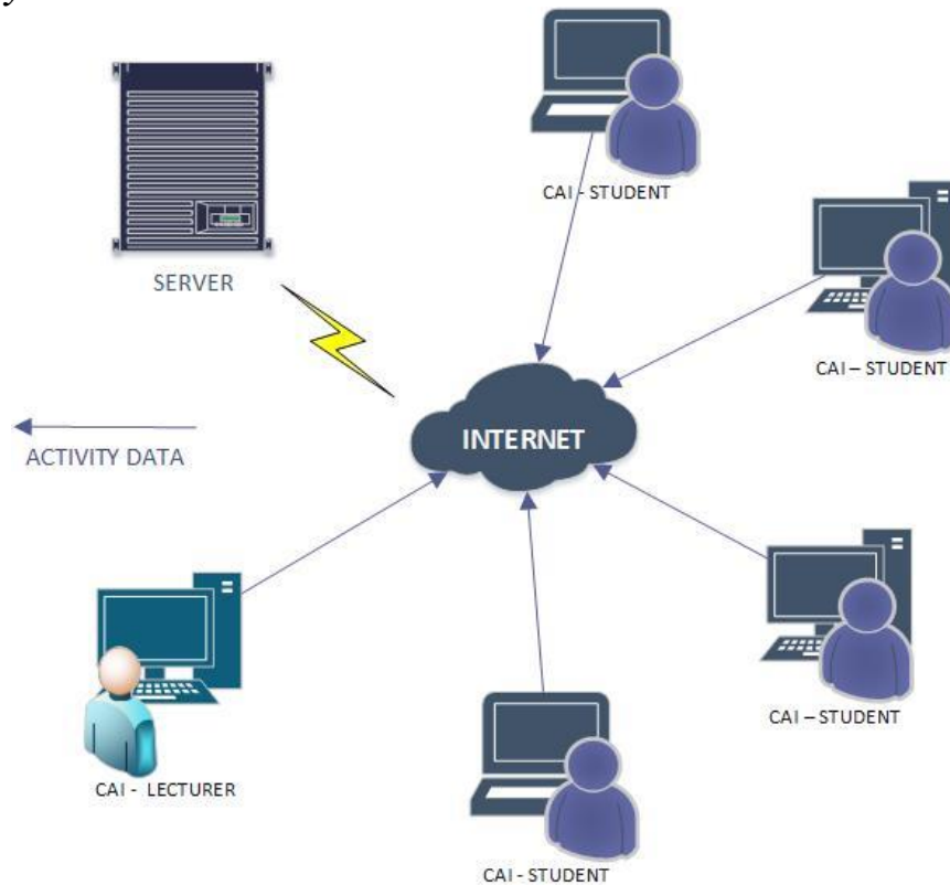
Gambar 1 Arsitektur CAI
