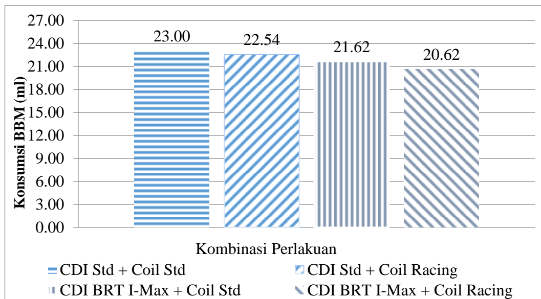
Gambar 4.12. Perbandingan Konsumsi Bahan Bakar Pengujian Torsi dan Daya
