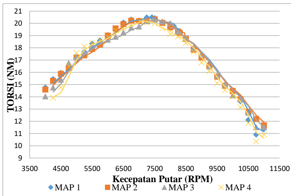
Gambar 4.5. Perbandingan Torsi dari Percobaan Mapping Variasi CDI BRT I-Max + Koil Standar + Busi Iridium
