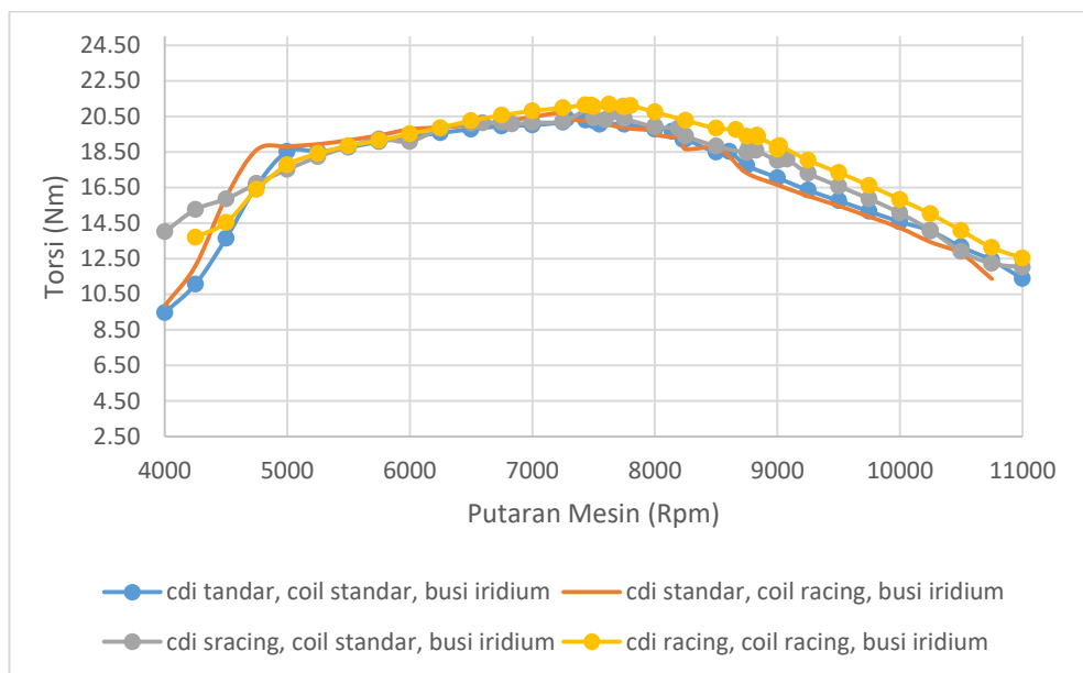
Gambar 4.9. Perbandingan Kecepatan Putar (rpm) dengan Torsi (N.m)
