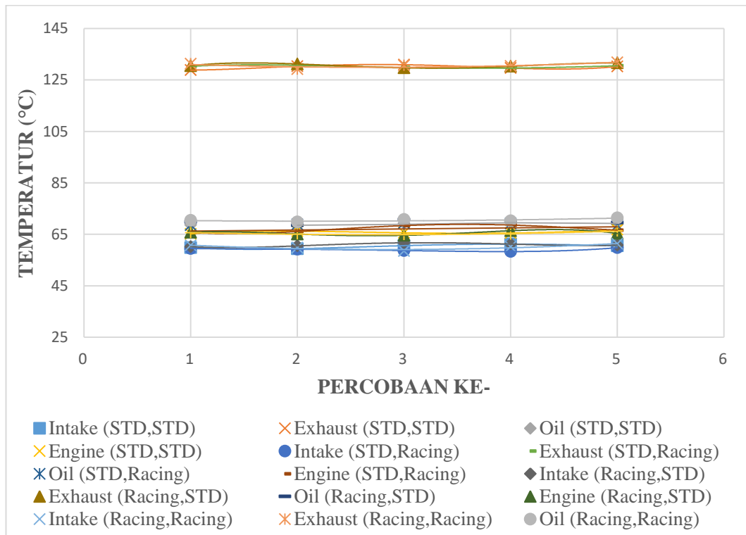
Gambar 4.14. Tempeartur Pengujian Konsumsi Bahan Bakar
