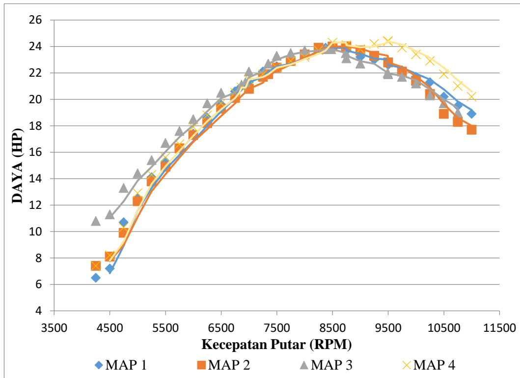
Gambar 4.7. Pebandingan Daya dari Percobaan Mapping Variasi CDI BRT I-Max + Koil TDR YZ + Busi iridium
