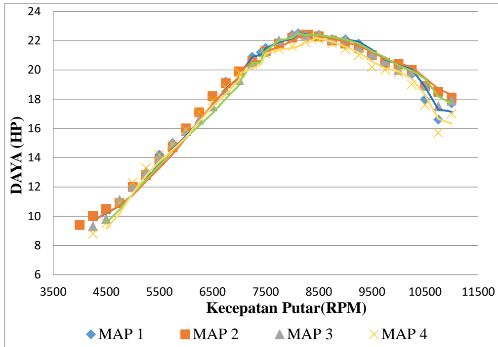
Gambar 4.4. Perbandingan Daya dari Percobaan Mapping Variasi CDI BRT I-Max + Koil Standar + Busi Iridium
