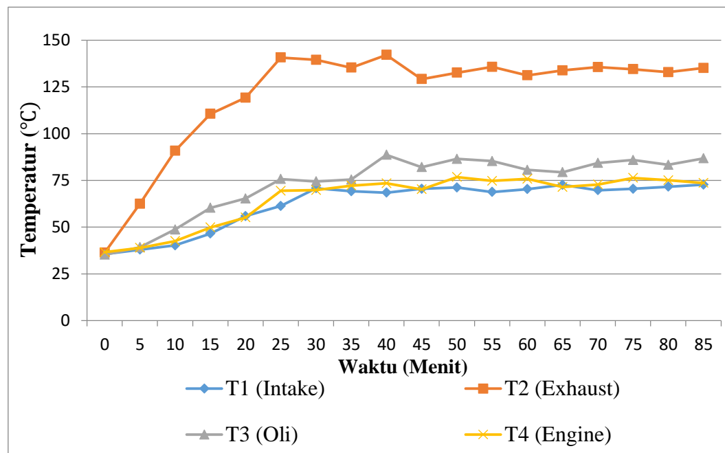
Gambar 4.2. Temperatur Kerja Sepeda Motor Scorpio z 225 cc
