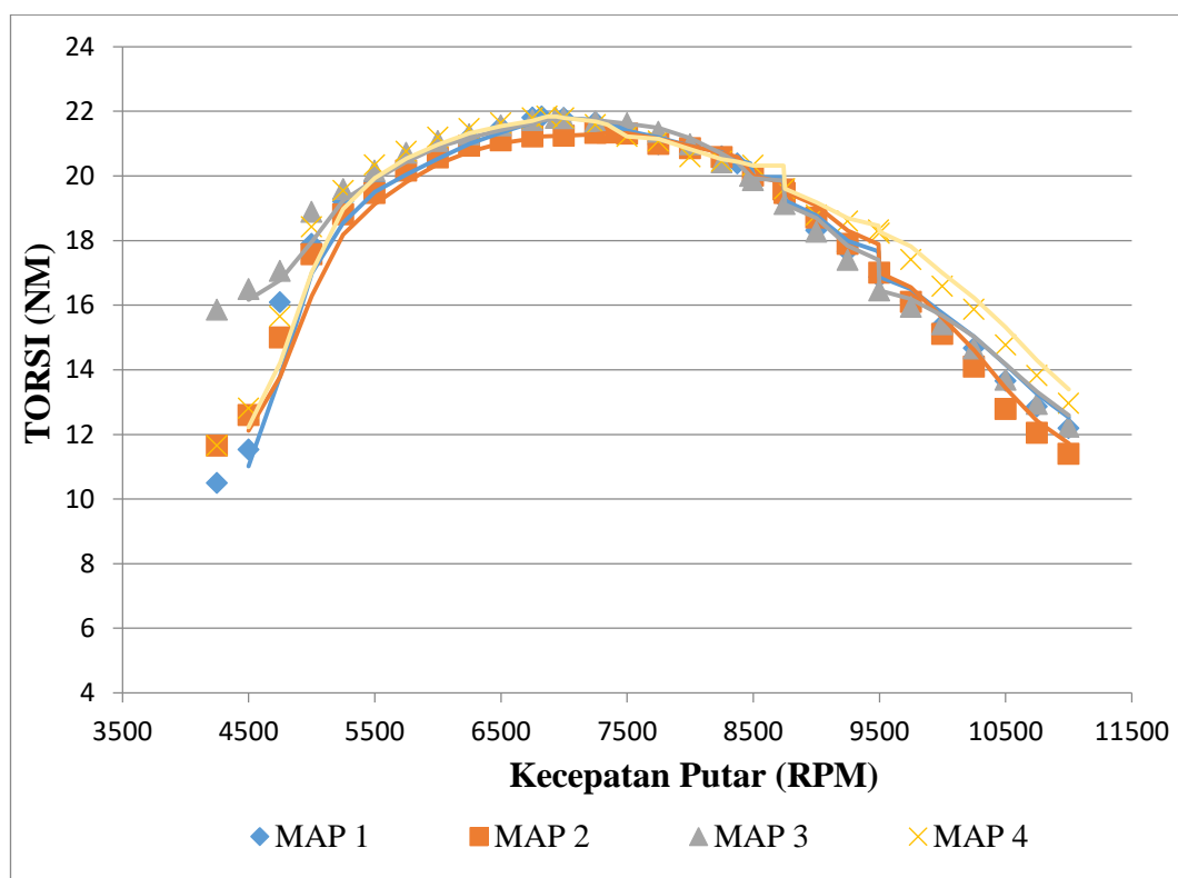
Gambar 4.8. Perbandingan Torsi dari Percobaan Mapping Variasi CDI BRT I-Max + Koil TDR YZ + Busi iridium
