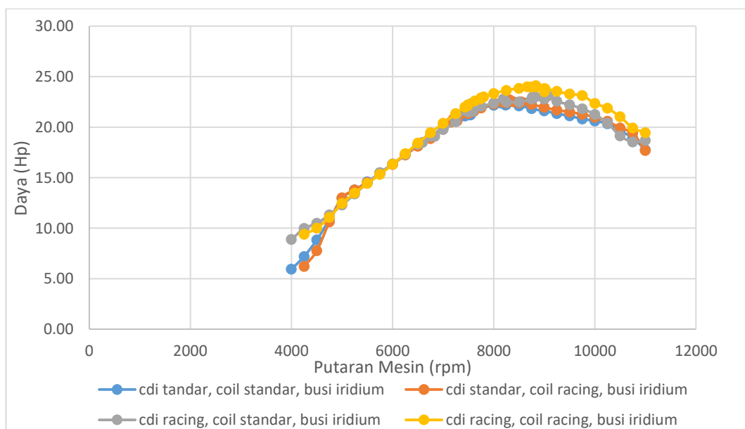
Gambar 4.10. Perbandingan Kecepatan Putar (rpm) dengan Daya (HP)
