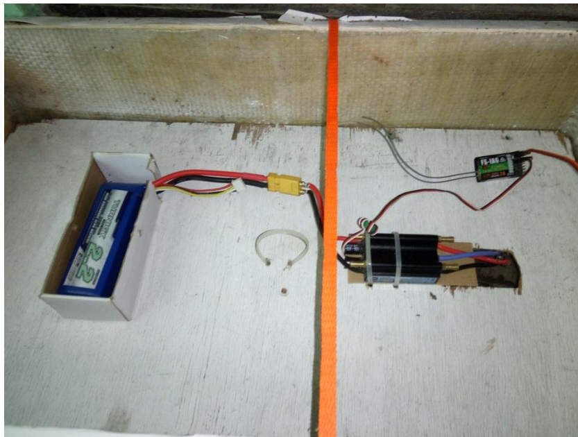
Gambar 1.4 Pemasangan Komponen Batrai Dan ESC
