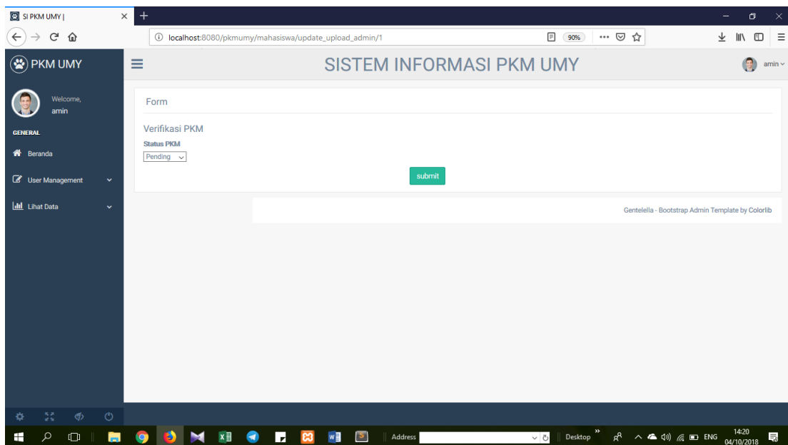
Gambar 4. 28 Halaman Verifikasi
