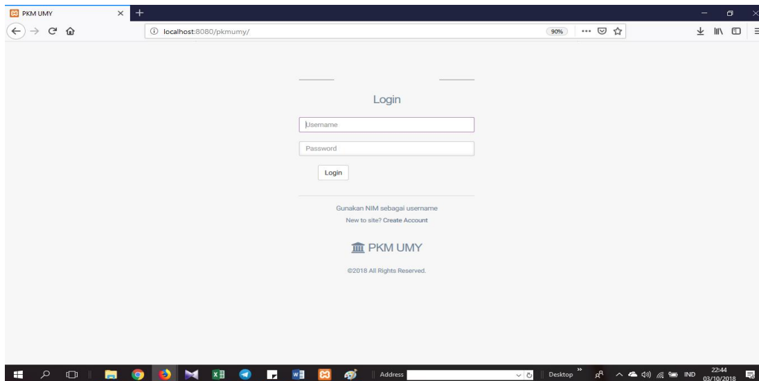
Gambar 4. 19 Halaman Login
