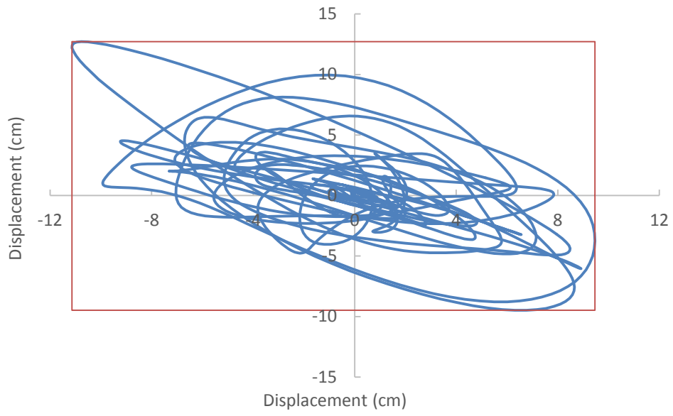
Lampiran 2. Grafik Obit of Top Displacement gedung tanpa Masonry dengan beban gempa Kobe
