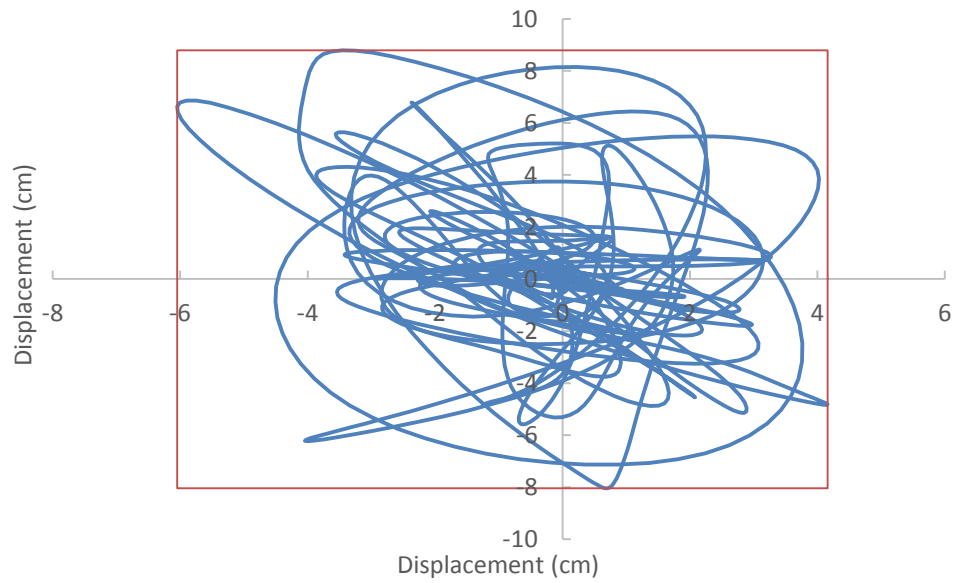
Lampiran 1. Grafik Obit of Top Displacement gedung dengan Masonry dengan beban gempa Kobe
