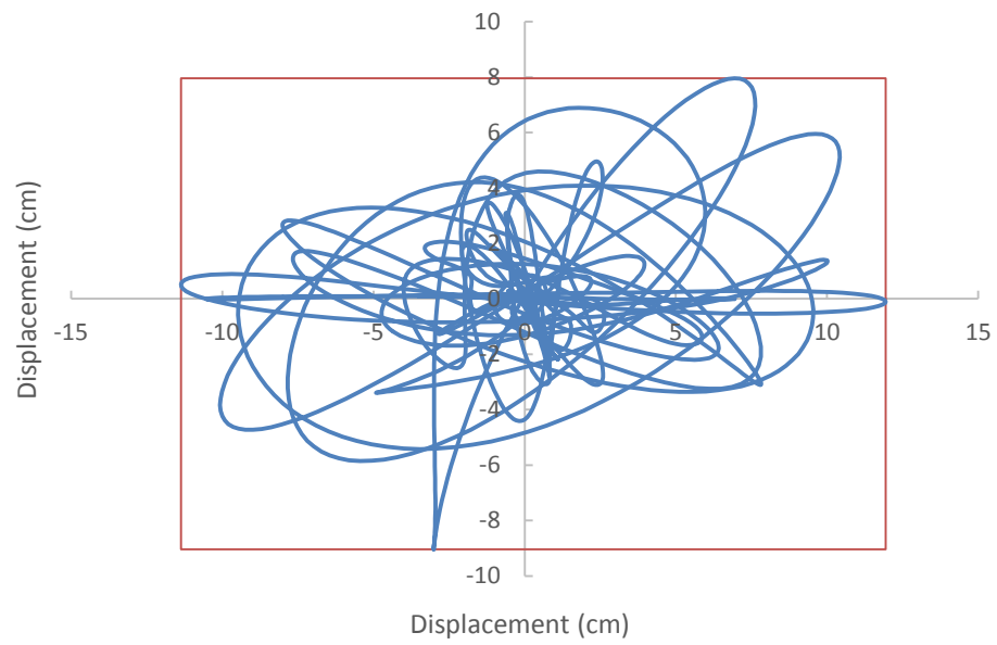
Lampiran 4. Grafik Obit of Top Displacement gedung tanpa Masonry dengan beban gempa Parkfield
