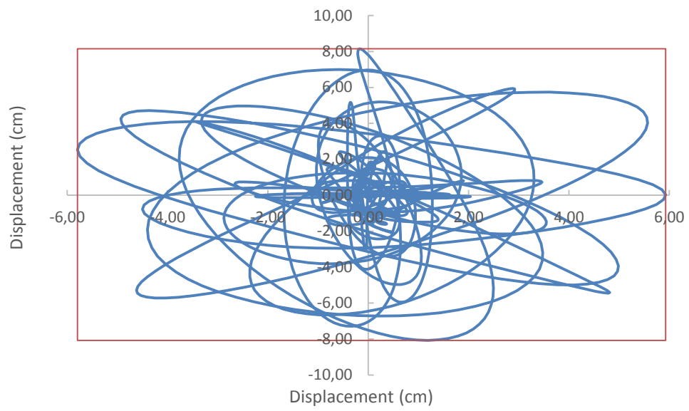
Lampiran 3. Grafik Obit of Top Displacement gedung dengan Masonry dengan beban gempa Parkfield
