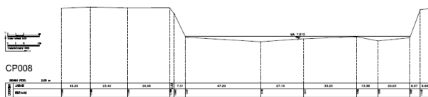
Gambar 6 Tampilan potongan melintang Sungai Progo Tengah bagian hilir (BBWS Serayu-Opak, 2017)
