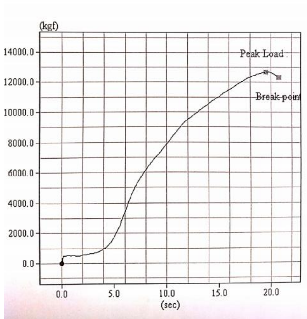
Gambar 20. Hubungan beban dan waktu pada benda uji 2 beton serat 6% 7 hari
