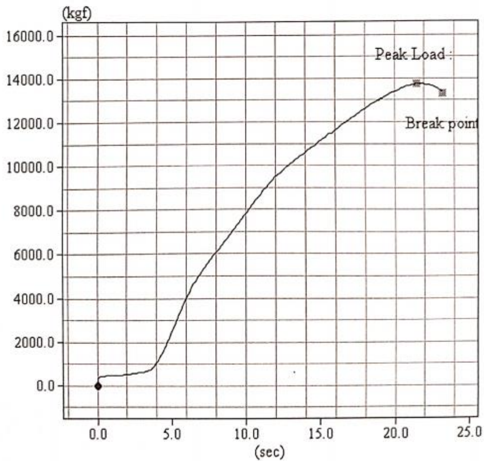
Gambar 21. Hubungan beban dan waktu pada benda uji 3 beton serat 6% 7 hari
