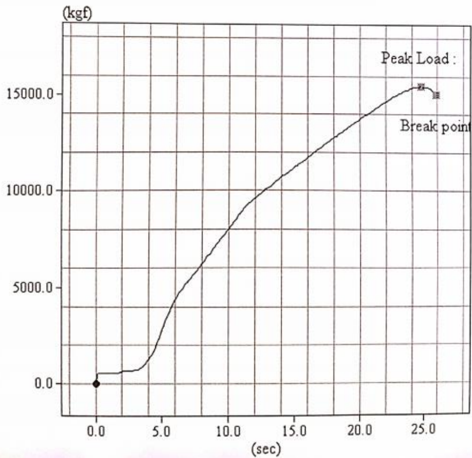
Gambar 14. Hubungan beban dan waktu pada benda uji 2 beton serat 4% 7 hari
