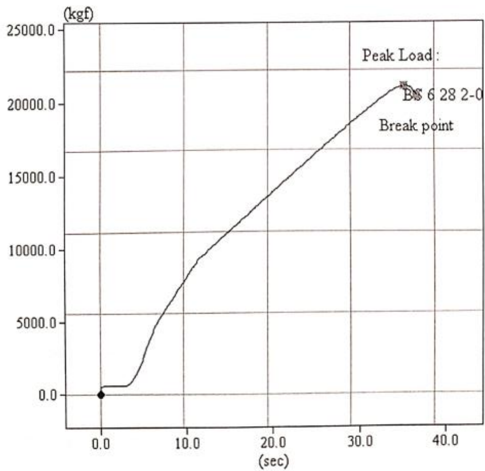
Gambar 23. Hubungan beban dan waktu pada benda uji 2 beton serat 6% 28 hari
