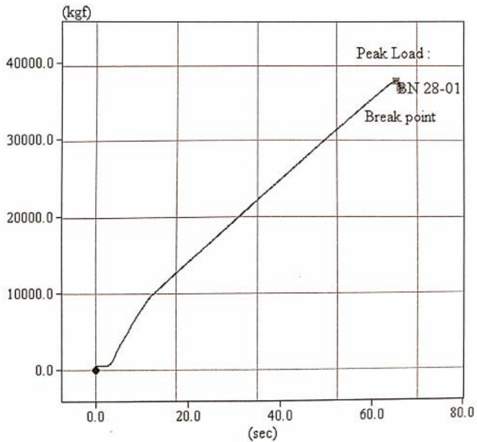
Gambar 4. Hubungan beban dan waktu pada benda uji 1 beton normal 28 hari
