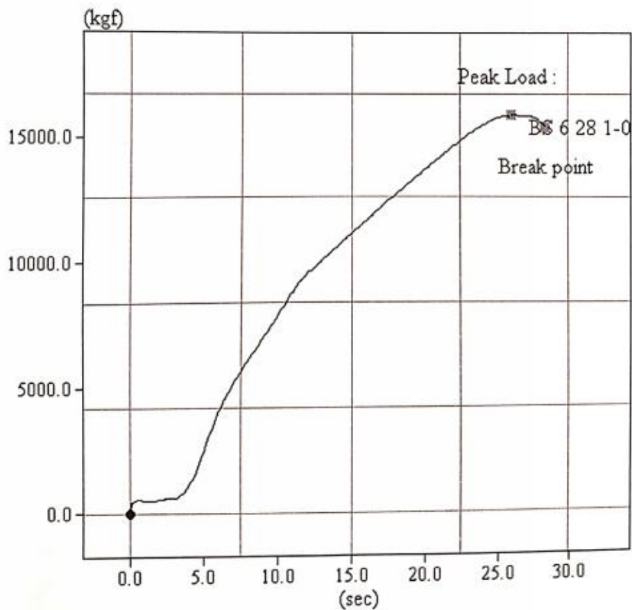
Gambar 22. Hubungan beban dan waktu pada benda uji 1 beton serat 6% 28 hari
