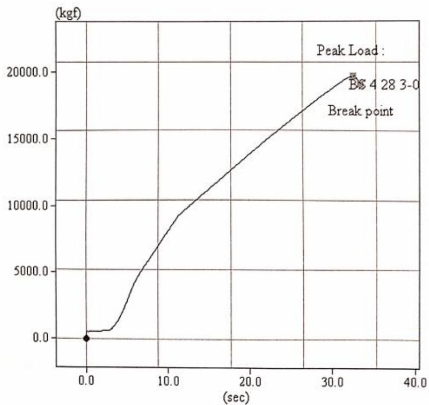
Gambar 18. Hubungan beban dan waktu pada benda uji 3 beton serat 4% 28 hari
