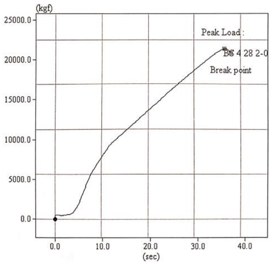
Gambar 17. Hubungan beban dan waktu pada benda uji 2 beton serat 4% 28 hari
