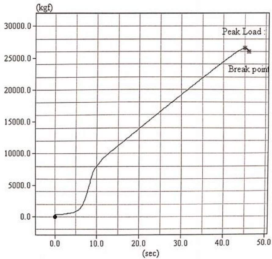
Gambar 11. Hubungan beban dan waktu pada benda uji 2 beton serat 2% 28 hari
