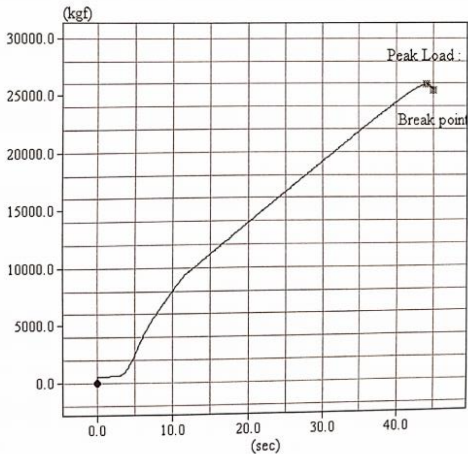
Gambar 12. Hubungan beban dan waktu pada benda uji 3 beton serat 2% 28 hari
