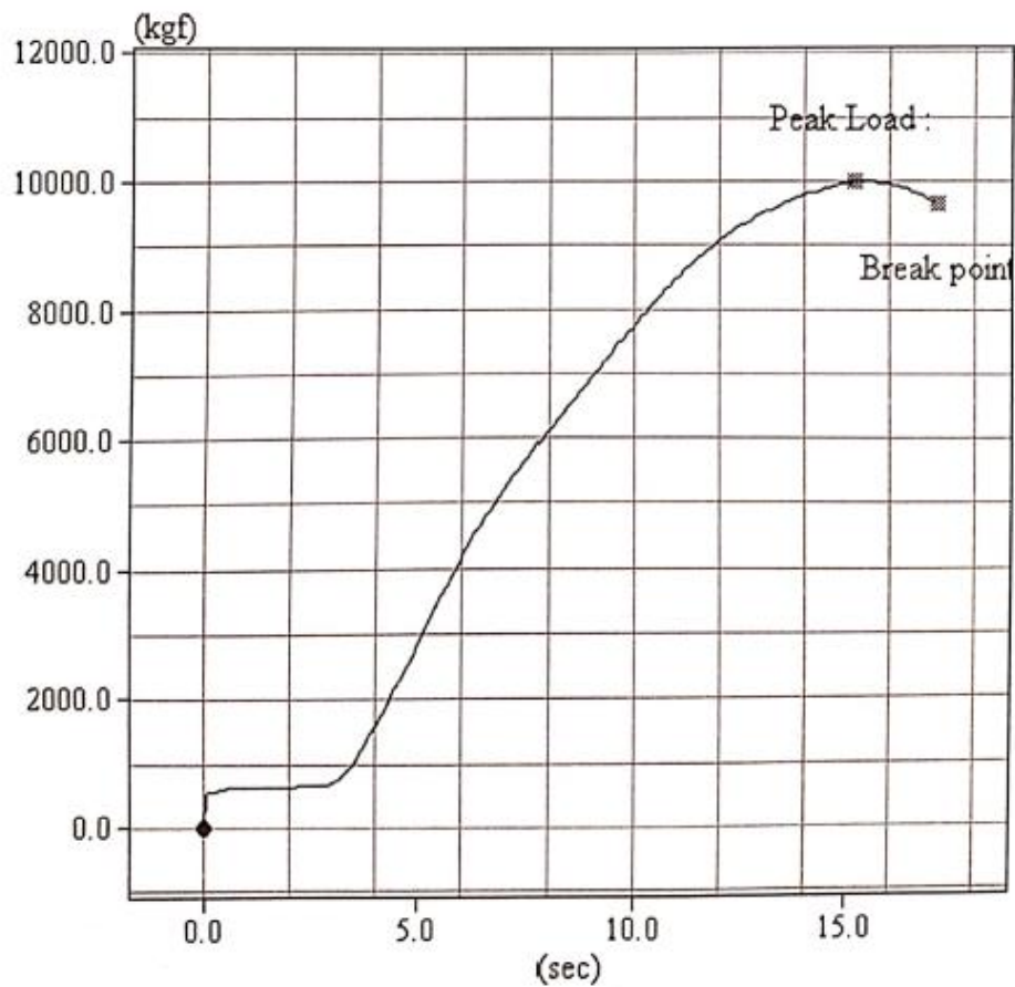
Gambar 19. Hubungan beban dan waktu pada benda uji 1 beton serat 6% 7 hari
