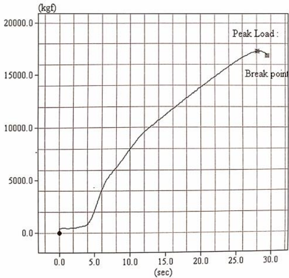
Gambar 9. Hubungan beban dan waktu pada benda uji 3 beton serat 2% 7 hari
