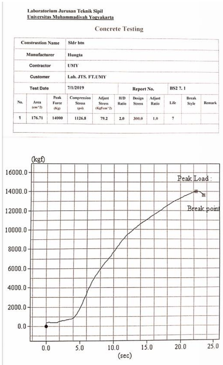
Gambar 7. Hubungan beban dan waktu pada benda uji 1 beton serat 2% 7 hari
