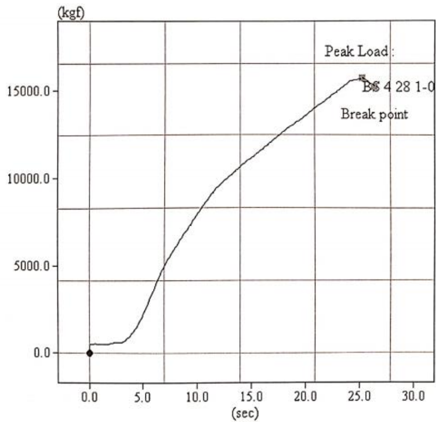
Gambar 16. Hubungan beban dan waktu pada benda uji 1 beton serat 4% 28 hari
