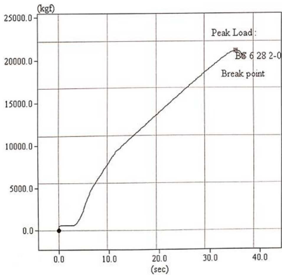
Gambar 24. Hubungan beban dan waktu pada benda uji 3 beton serat 6% 28 hari
