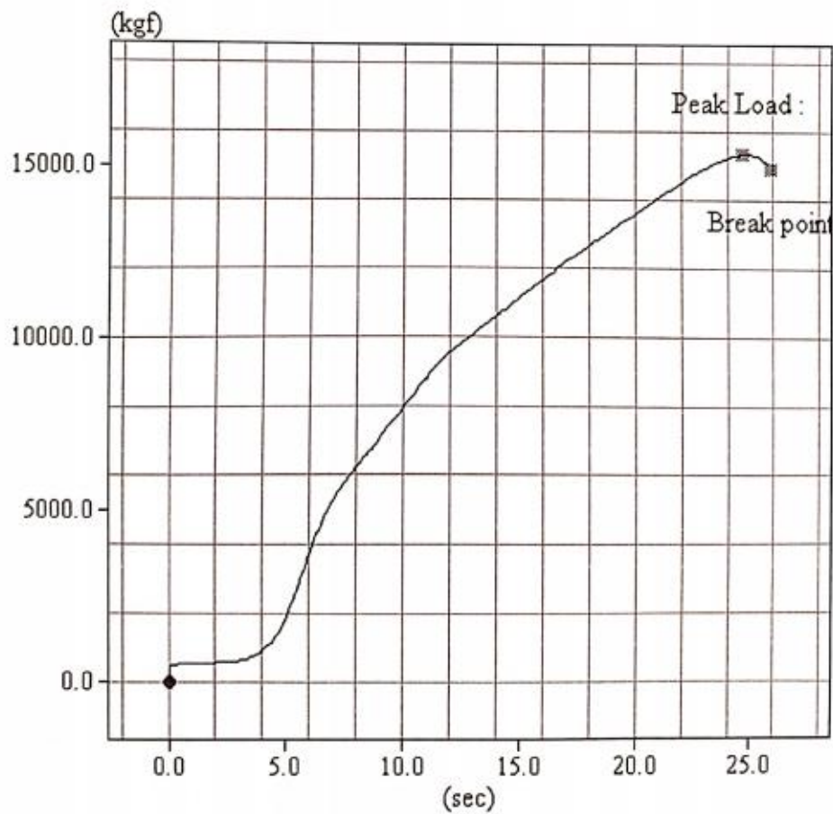
Gambar 13. Hubungan beban dan waktu pada benda uji 1 beton serat 4% 7 hari
