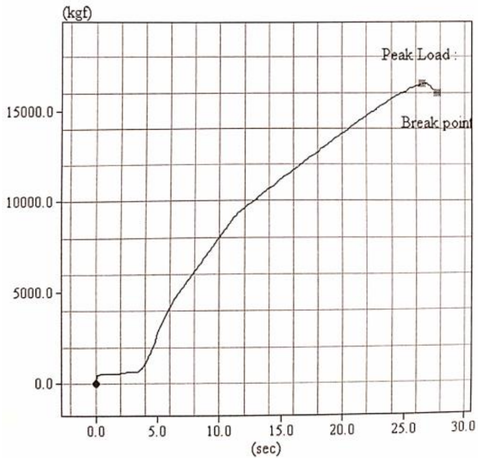
Gambar 8. Hubungan beban dan waktu pada benda uji 2 beton serat 2% 7 hari
