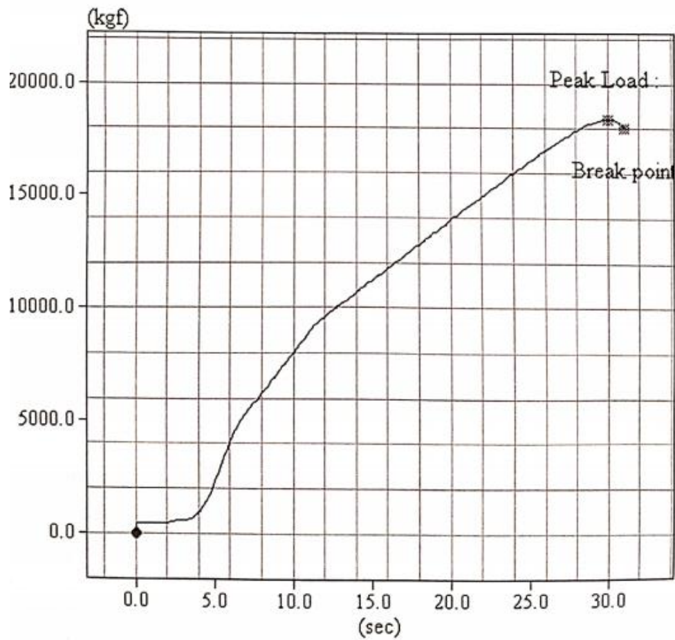
Gambar 1. Hubungan beban dan waktu pada benda uji 1 beton normal 7 hari
