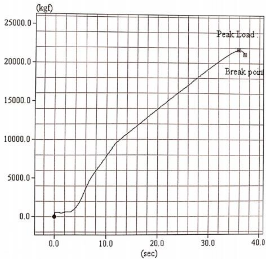
Gambar 10. Hubungan beban dan waktu pada benda uji 1 beton serat 2% 28 hari
