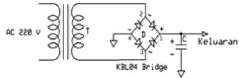
GAMBAR 5. Skema rangkaian power supply
