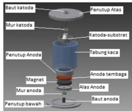
GAMBAR 3. Desain komponen vacuum chamber
