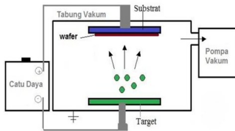
GAMBAR 2. Skema Mesin Sputtering
