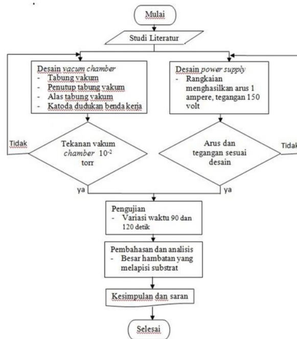
GAMBAR 1. Alur perancangan dan pembuatan mesin sputtering
