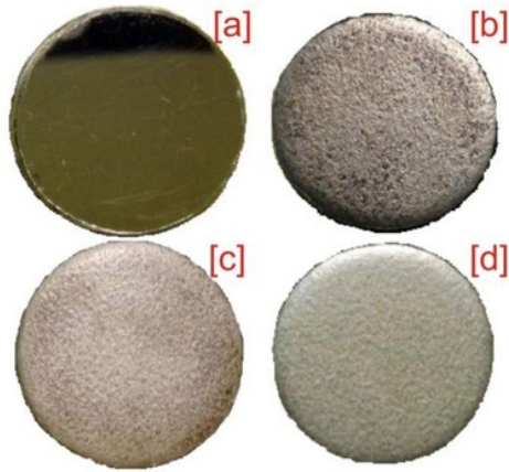
Gambar 3. [a] Tanpa perlakuan shot peening , perlakuan shot peening diameter steel ball [b] 0,4 mm, [c] 0,6 mm, [d] 0,7 mm.
