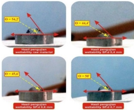
Gambar 9. Uji wettability spesimen SS AISI 304
