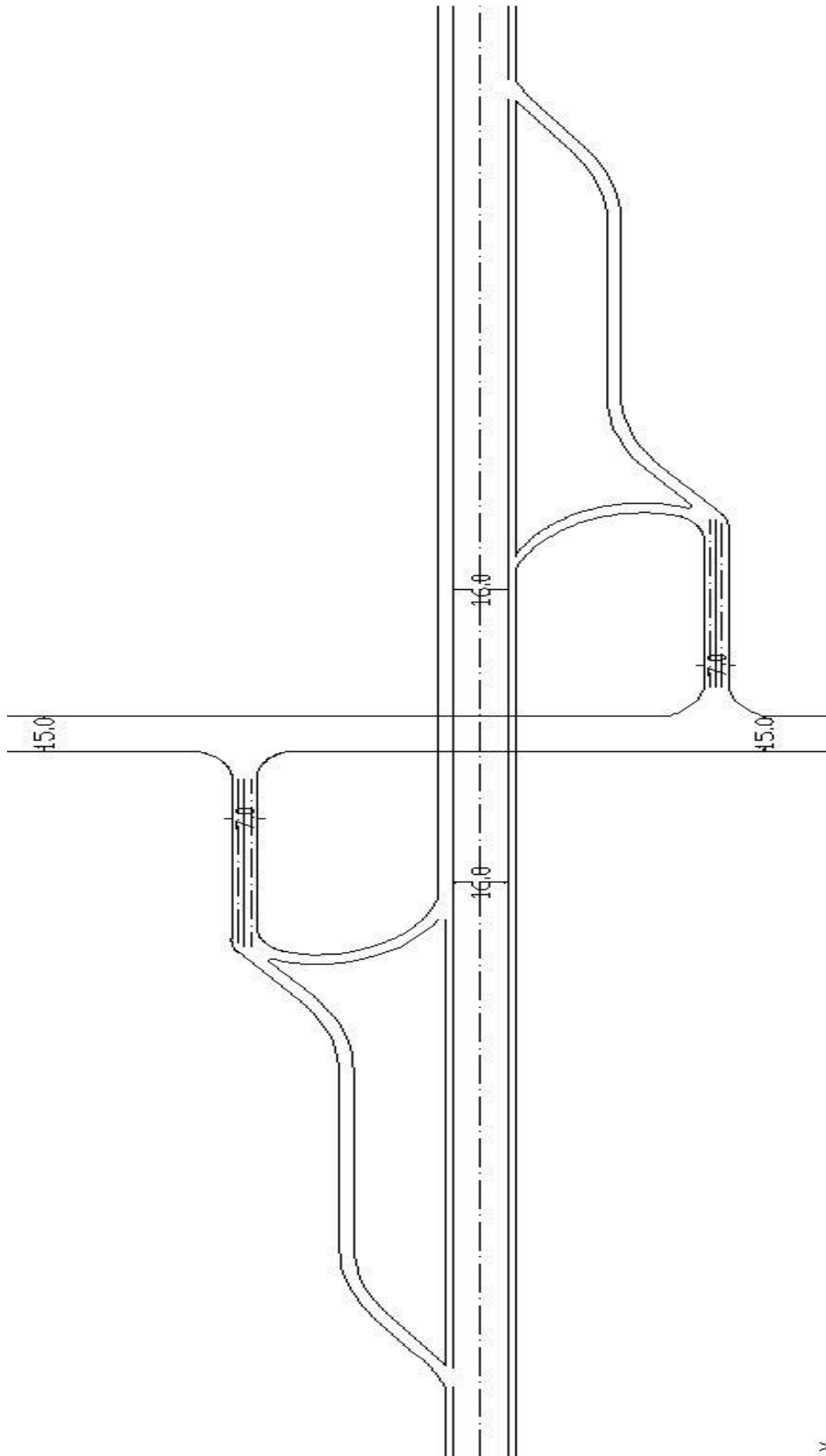
Lampiran 2. Desain Geometrik Simpang Parclo B2 default
