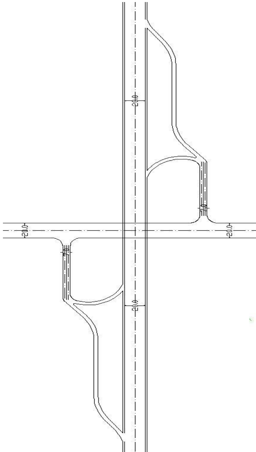
Lampiran 3. Desain geometrik Simpang Parclo B2 modifikasi
