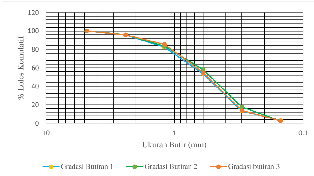
Gambar 1. Hubungan antara % lolos kumulatif dan ukuran butir agregat
