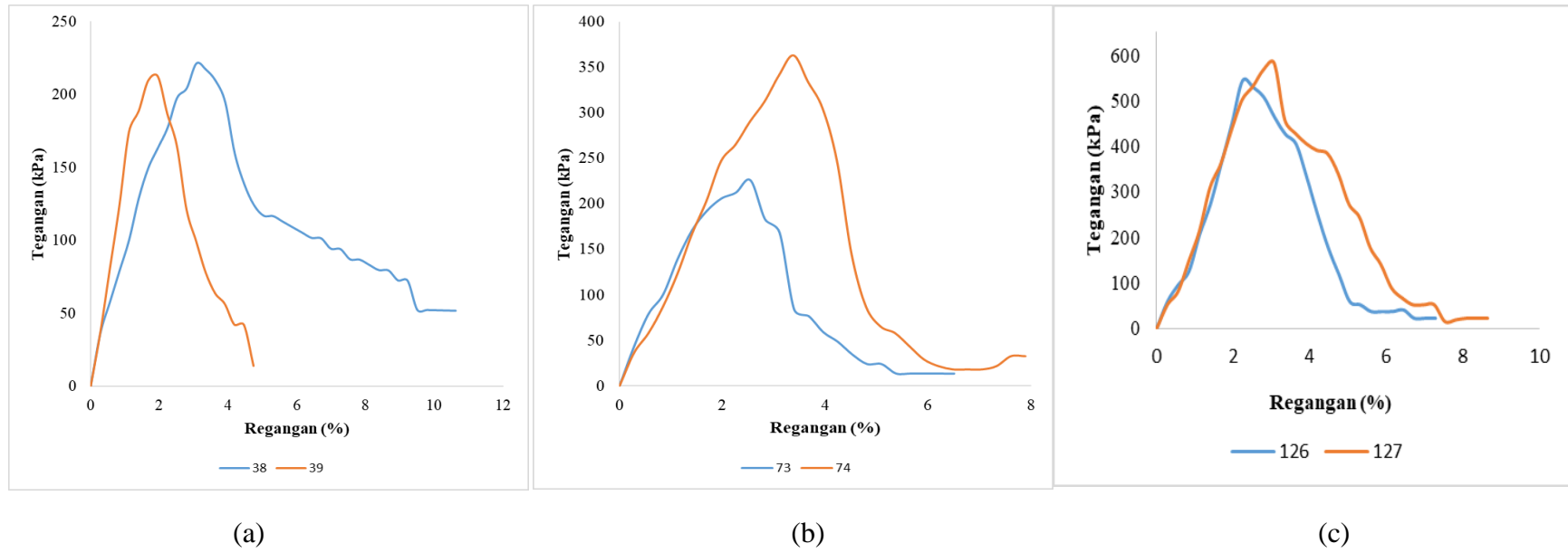
Gambar 6 (a) kondisi ODM (b) kondisi OMC (c) kondisi OWM
