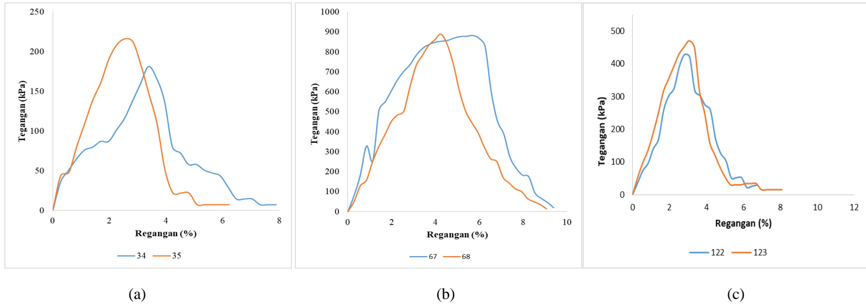
Gambar 8 (a) kondisi ODM (b) kondisi OMC (c) kondisi OWM
