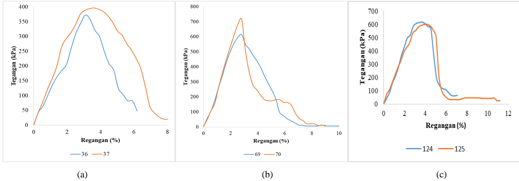
Gambar 7 (a) kondisi ODM (b) kondisi OMC (c) kondisi OWM
