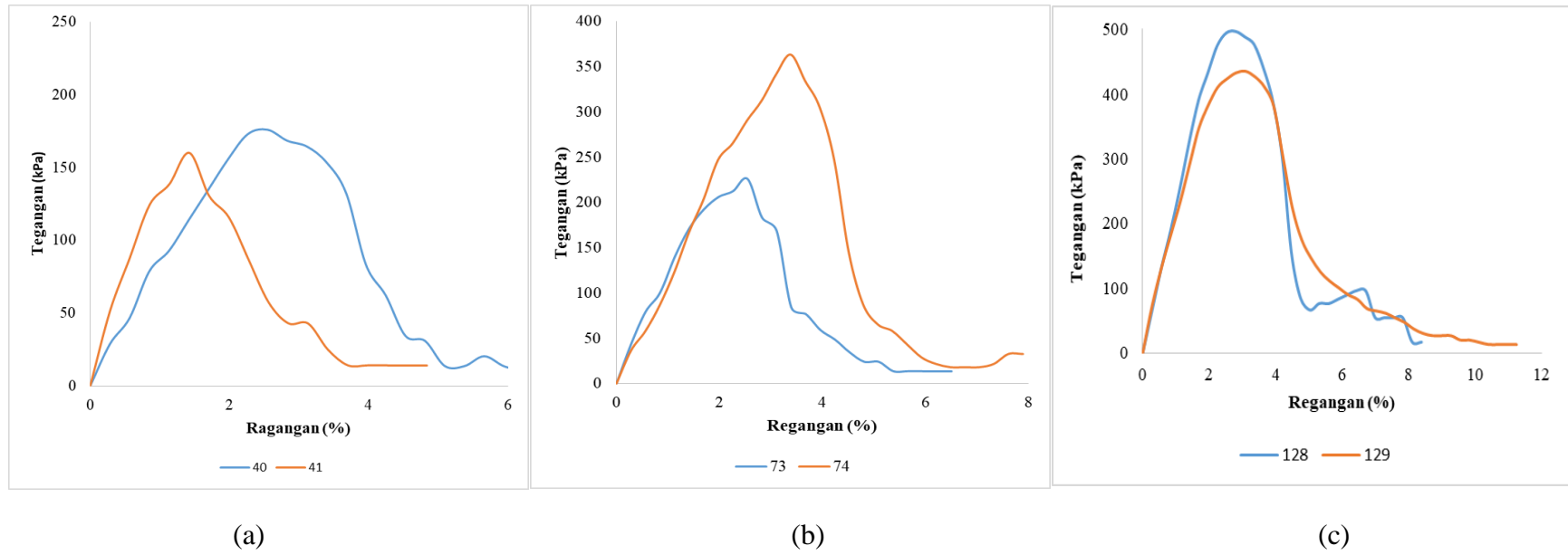
Gambar 5 (a) kondisi ODM (b) kondisi OMC (c) kondisi OWM
