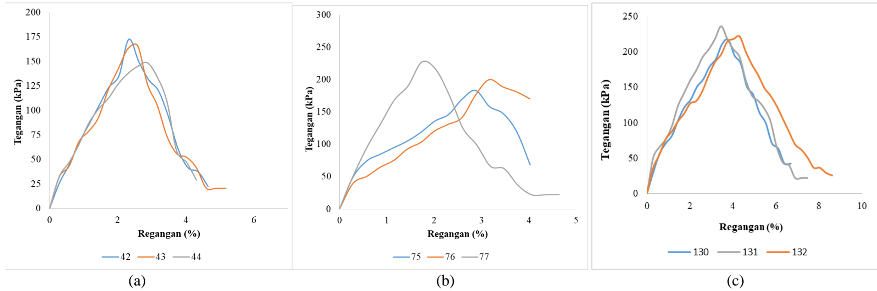
Gambar 4 (a) kondisi ODM (b) kondisi OMC (c) kondisi OWM
