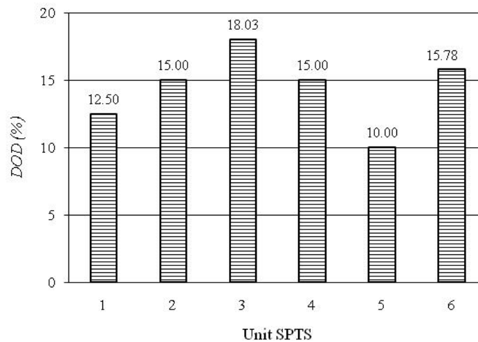
GAMBAR 7. DOD baterai
