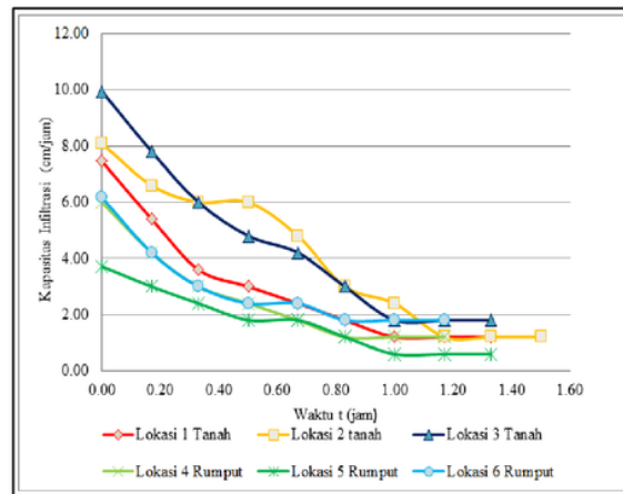
Gambar 4. Grafik kapasitas infiltrasi Lokasi 1 sampai Lokasi 6
