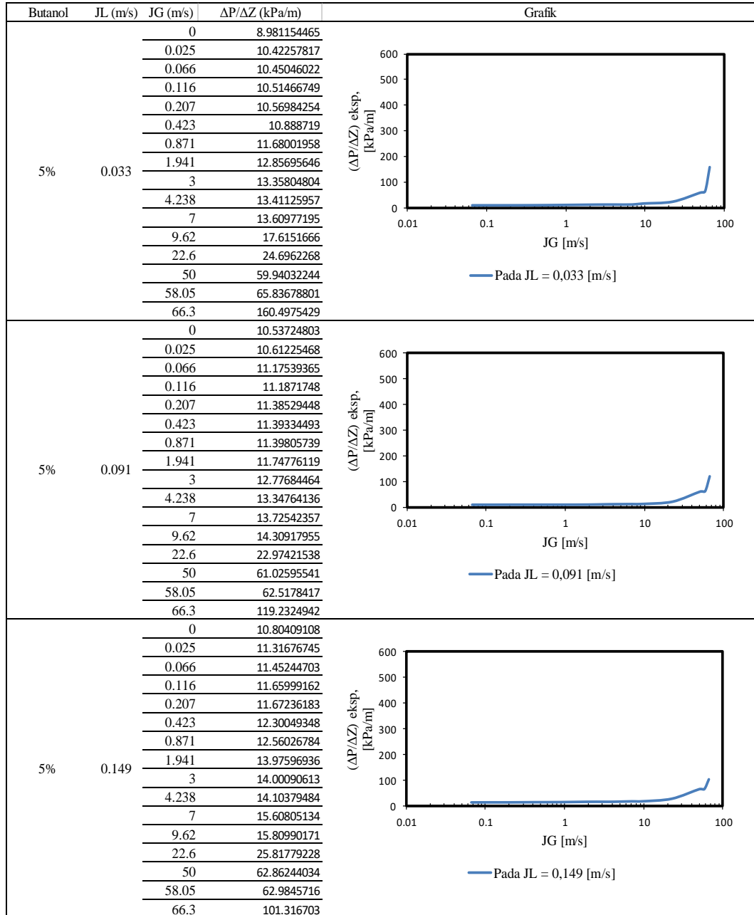
Lampiran 1 Tabel Variasi Kecepatan Superfisial Gas ( J_G ) Terhadap Gradien Tekanan Pada Butanol 5%
