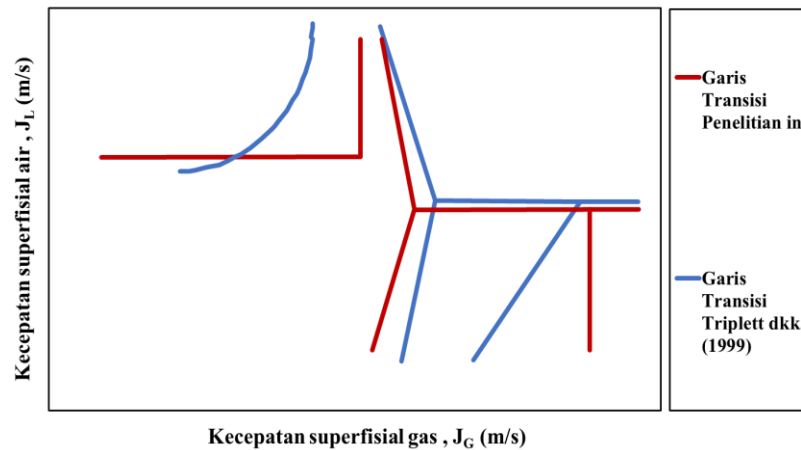
Gambar 8. Perbandingan peta pola aliran dengan penelitian terdahulu
