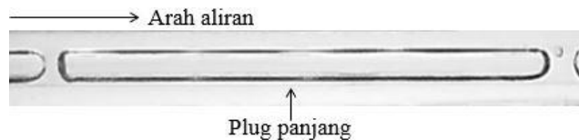
Gambar 2. Pola aliran plug pada J_G = 0,207 m/s, J_L = 0,091 m/s
