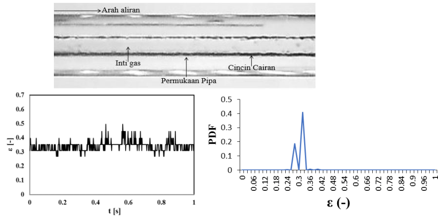
Gambar 12. Pola aliran annular , time average, dan PDF pada J_G = 58,05 m/s, J_L = 0,033 m/s
