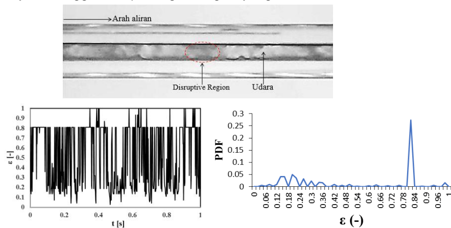
Gambar 13. Pola aliran churn , time average, dan PDF pada J_G = 22,6 m/s, J_L = 0,539 m/s
