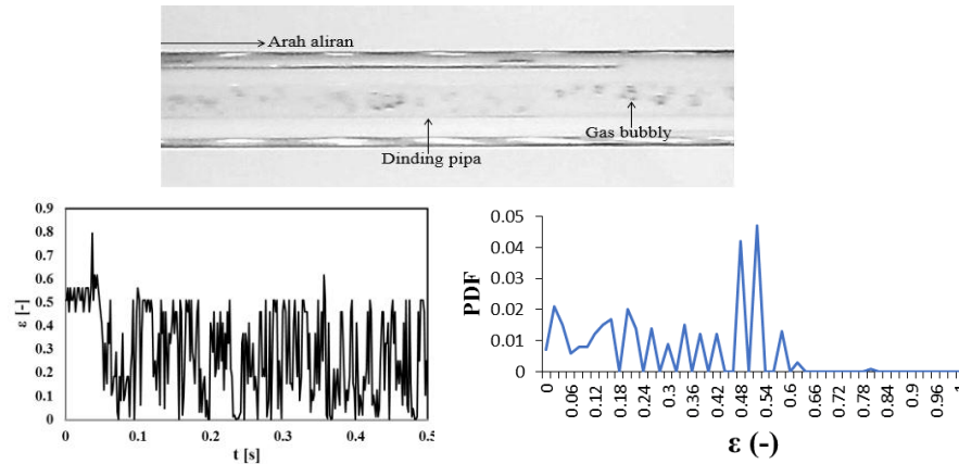
Gambar 10. Pola aliran bubbly , time average dan PDF pada J_G = 0,066 m/s, J_L = 2,297 m/s
