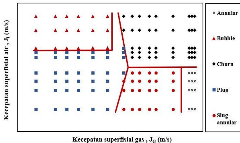
Gambar 7. Peta pola aliran
