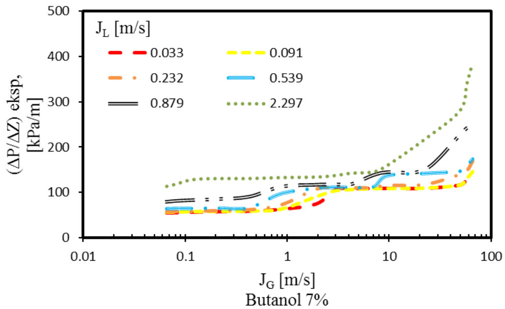
Gambar 14. Pengaruh J_L terhadap gradien tekanan dengan variasi J_G ,
