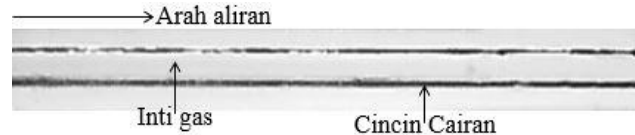
Gambar 5. Pola aliran annular pada J_G = 66,3 m/s, J_L = 0,091 m/s
