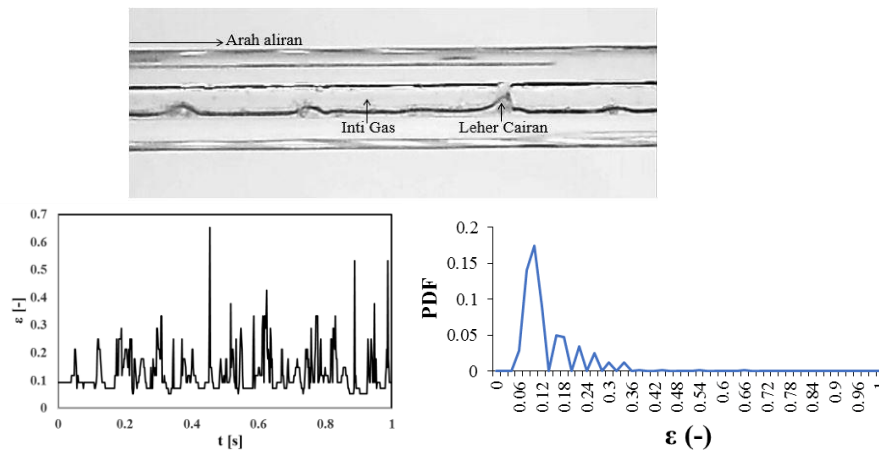
Gambar 11. Pola aliran slug annular , time average, dan PDF pada J_G = 4,238 m/s, J_L = 0,033 m/s
