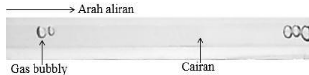
Gambar 3. Pola aliran bubbly pada J_G = 0,066 m/s, J_L = 0,879 m/s
