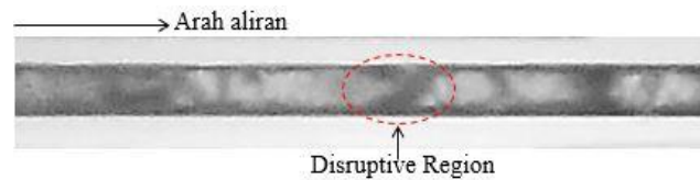
Gambar 6. Pola aliran churn pada J_G = 22,6 m/s, J_L = 0,879 m/s
