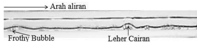
Gambar 4. Pola aliran slug-annular pada J_G = 3 m/s, J_L = 0,091 m/s
