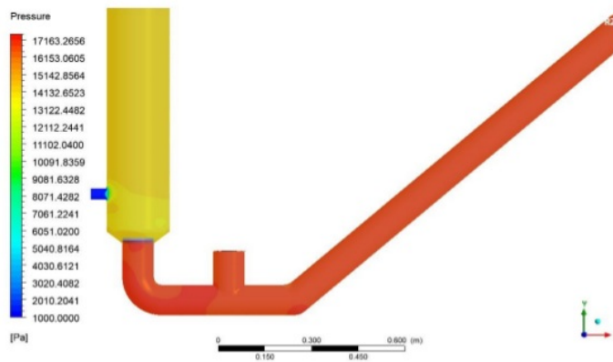
Gambar 3.2 Kontur tekanan pada Kondisi Katup Pengantar Terbuka 8 cm
