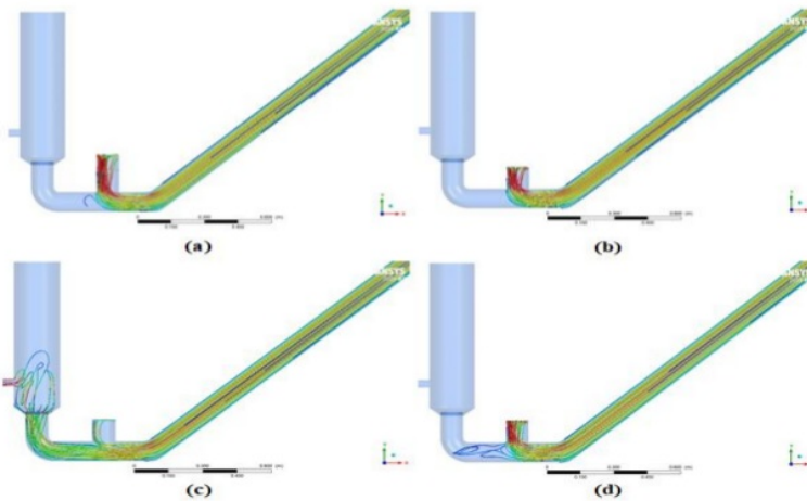
Gambar 3.4 Kontur streamline pada saat (a). Katup buang terbuka 8 cm, (b). Katup buang tertutup 8 cm, (c). Katup pengantar terbuka 1 cm, (d). Katup pengantar tertutup 1 cm.
