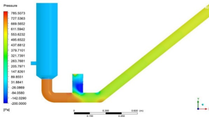
Gambar 3.1 Kontur tekanan pada tabung kondisi katup buang terbuka 8 cm
