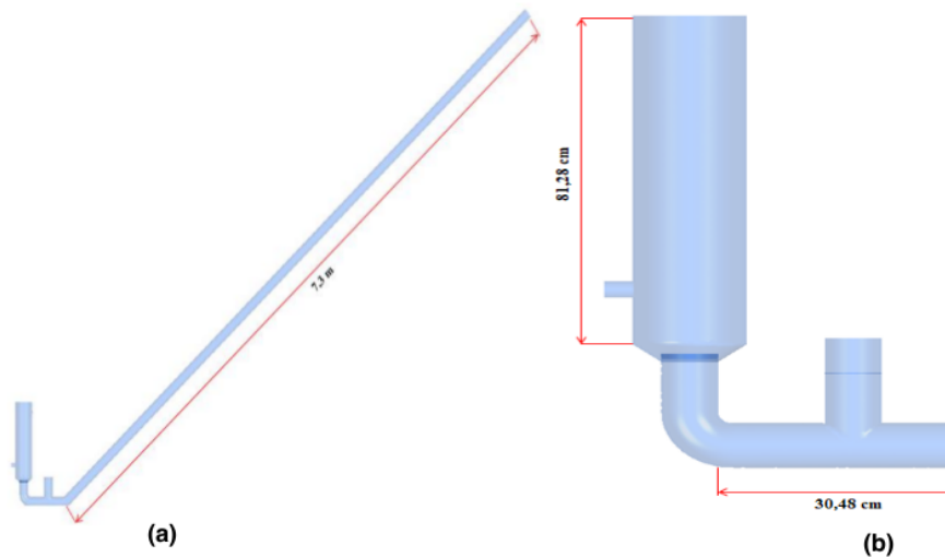
Gambar 2.1 (a). Geometri Pompa Hydrum dan Pipa Pesat, (b). Geometri Pompa Hydrum
