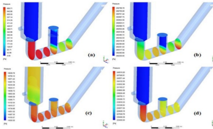
Gambar 3.6 Kontur kecepatan pada saat (a). Katup buang terbuka 8 cm, (b). Katup buang tertutup 8 cm, (c). Katup pengantar terbuka 1 cm, (d). Katup pengantar tertutup 1 cm.
