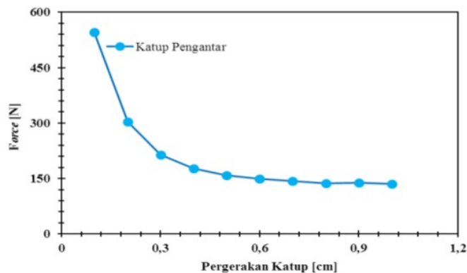
Gambar 3.7 Hubungan antara Force dan Pergerakan Katup Pengantar
