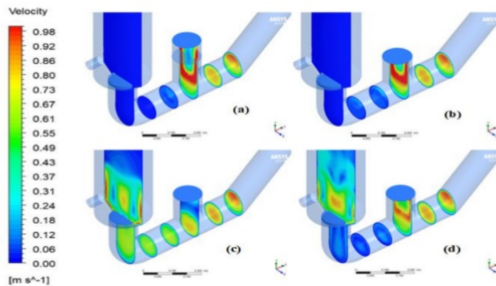
Gambar 3.5 Kontur kecepatan pada kondisi (a). Katup buang terbuka 8 cm, (b). Katup buang tertutup 8 cm, (c). Katup pengantar terbuka 1 cm, (d). Katup pengantar tertutup 1 cm.
