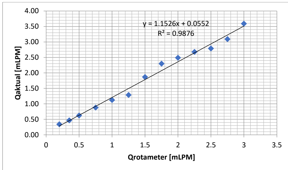
Lampiran 25. Grafik dan tabel terkalibrasi rotameter air
