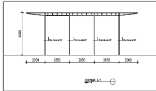
D. Potongan Y-Y
