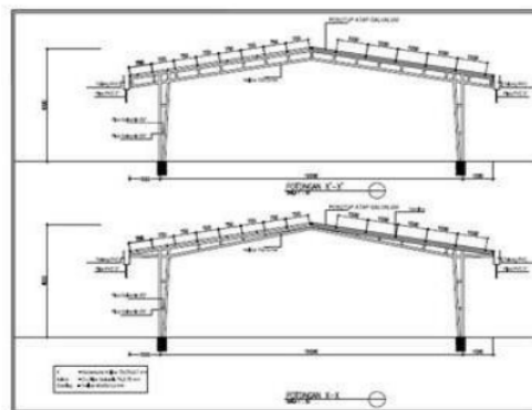
C. Potongan X-X dan X'-X'
