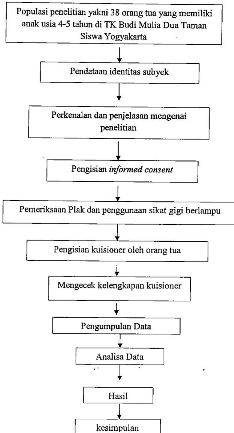
Gambar 3 : Alur penelitian
