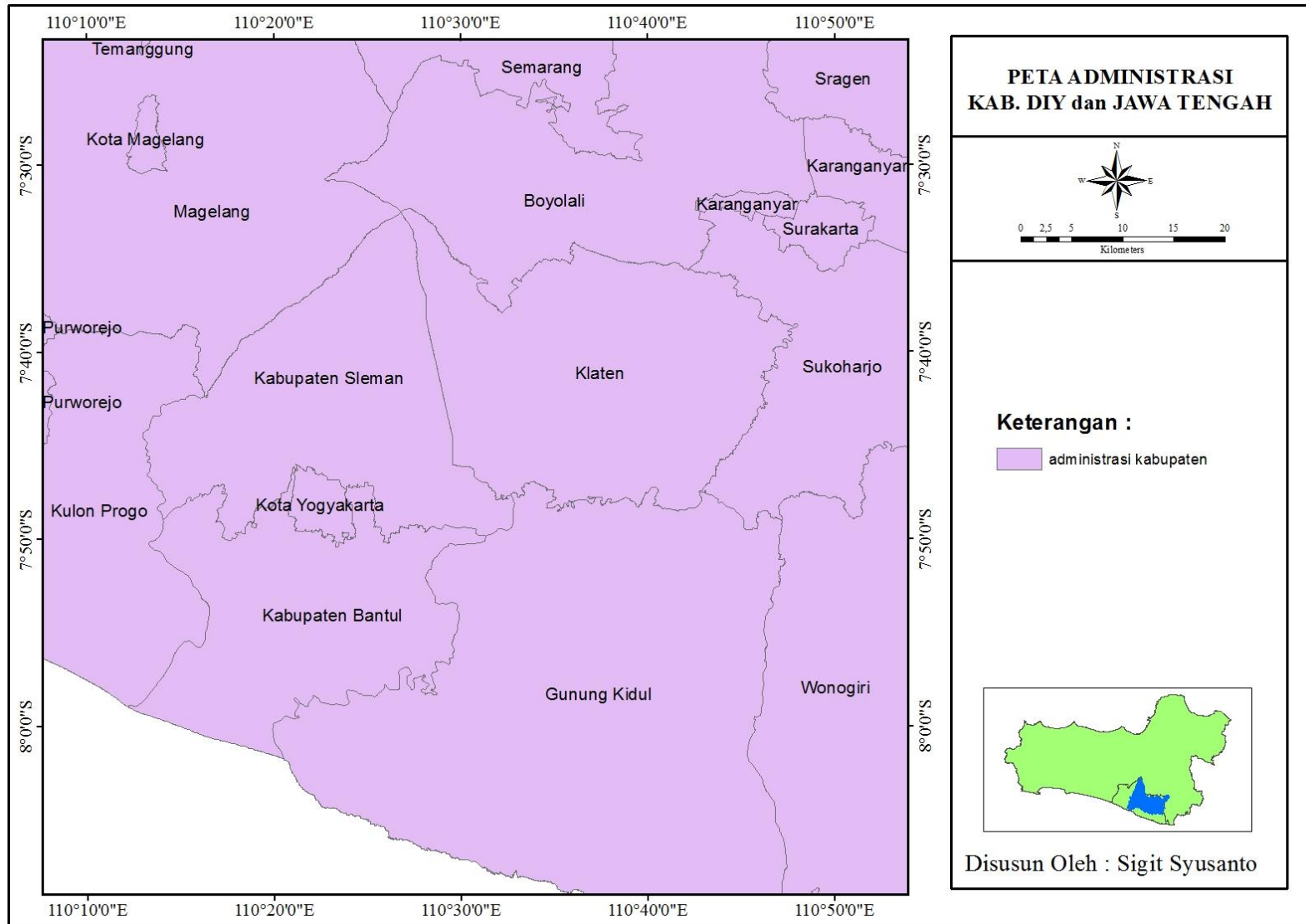
Gambar 3. Peta Administrasi Dari Badan Informasi Geospasial (BIG)
