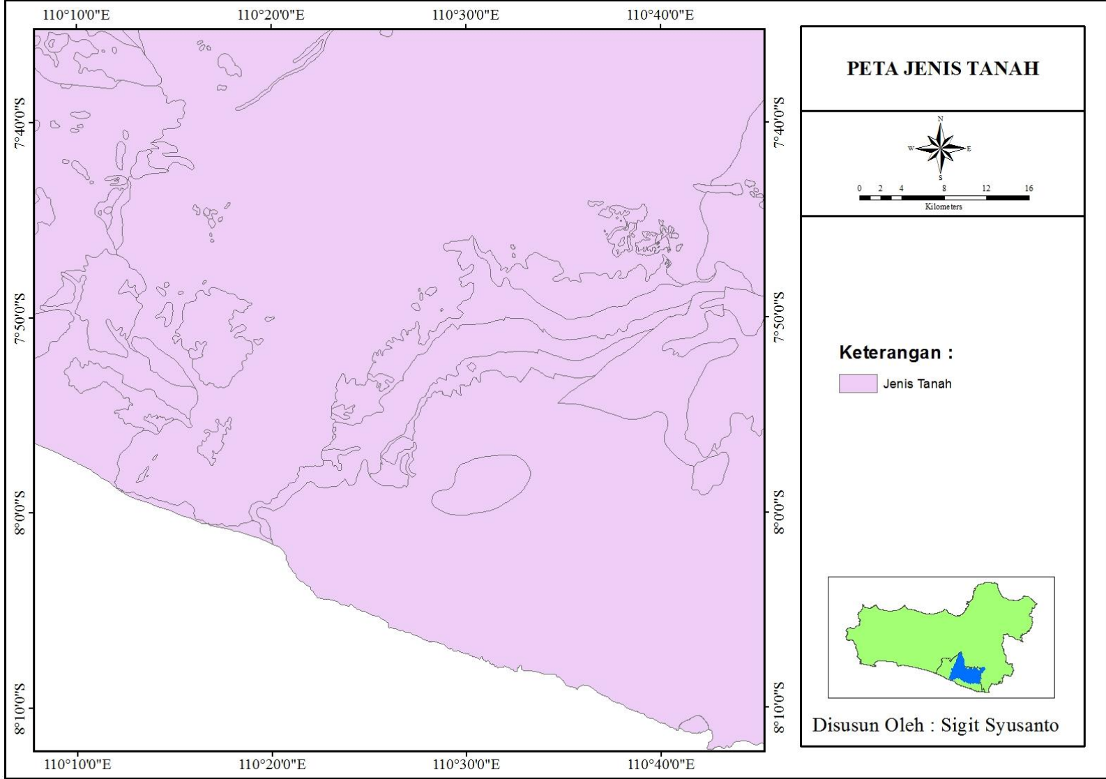
Gambar 5. Peta Jenis Tanah Dari Badan Informasi Geospasial (BIG)
