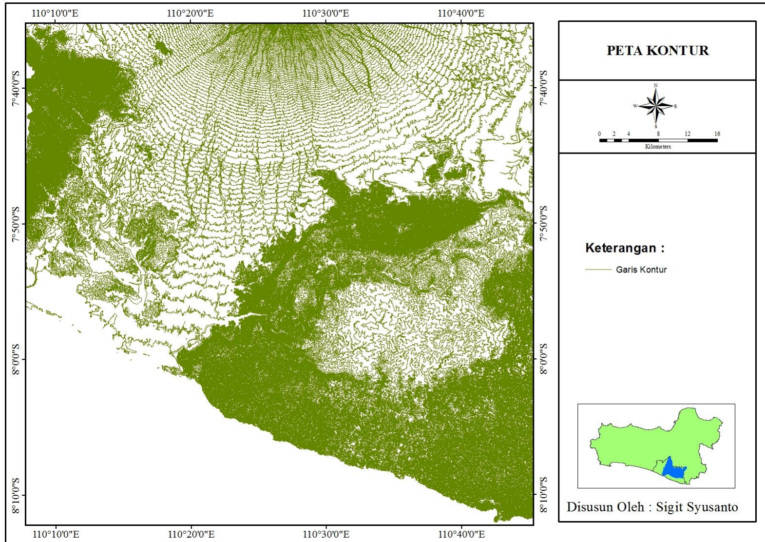
Gambar 2. Peta Kontur Dari Badan Informasi Geospasial (BIG)
