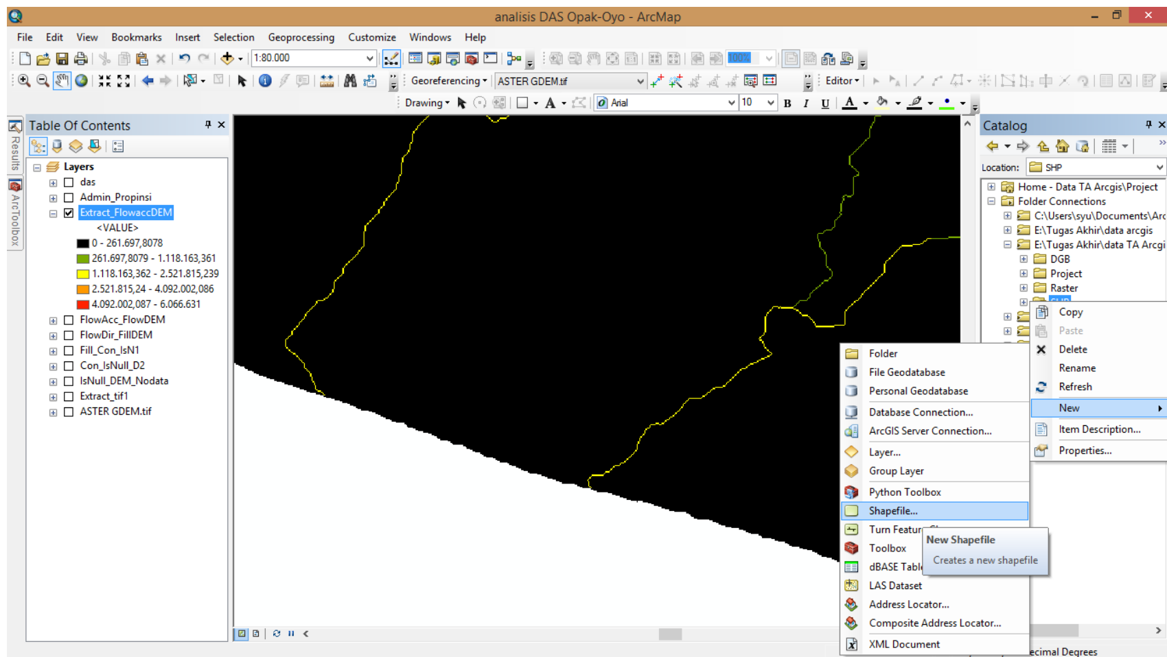
Gambar 12. Penentuan Titik Outlet
