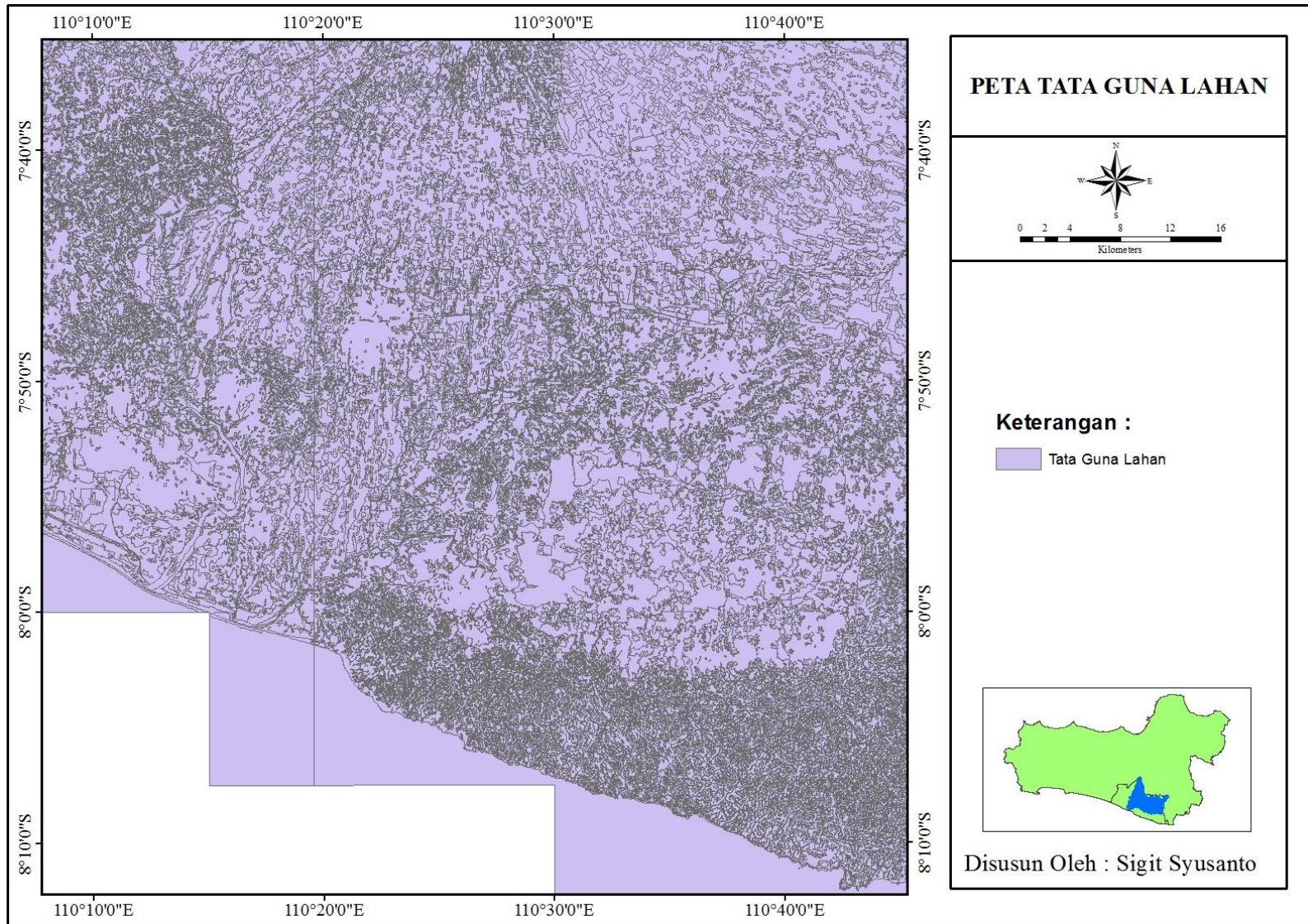
Gambar 4. Peta Tata Guna Lahan Dari Badan Informasi Geospasial (BIG)
