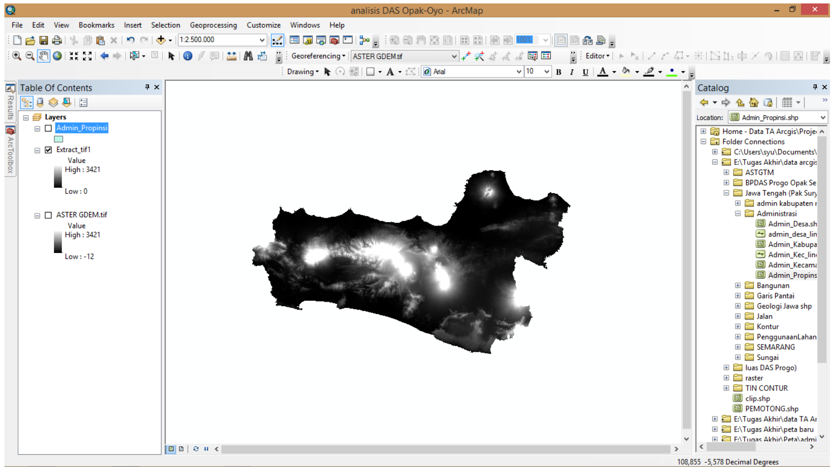
Gambar 8. Hasil Pemotongan DEM.
