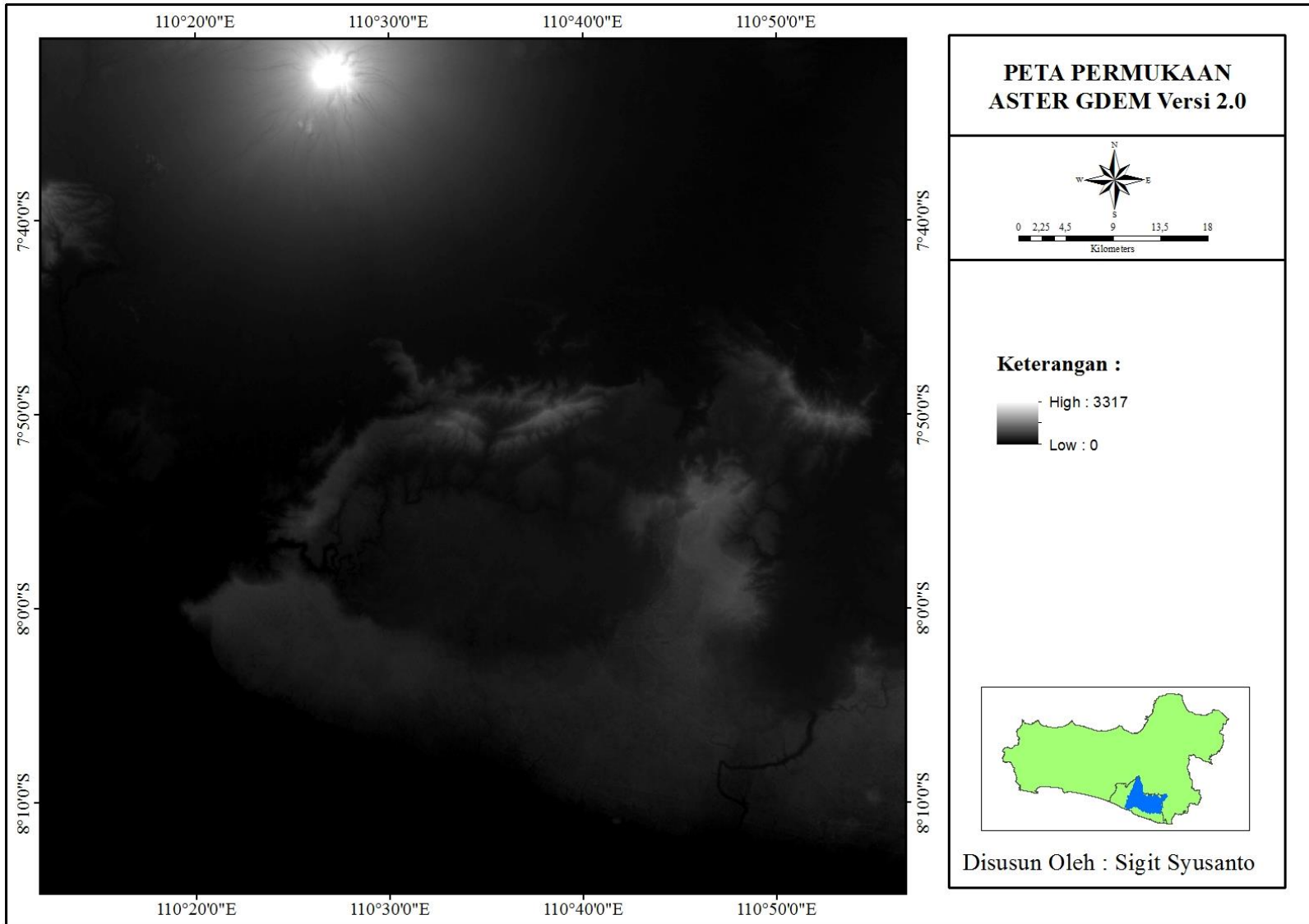
Gambar 1. Peta Permukaan ASTER GDEM V 2.0
