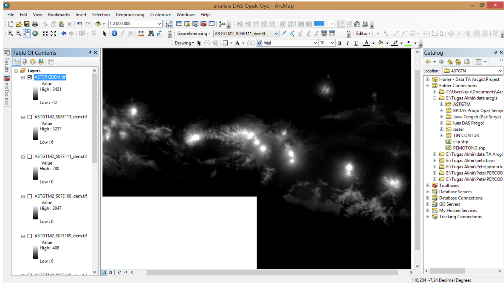
Gambar 7. Hasil Penggabungan Peta DEM ASTER GDEM V 2.0
