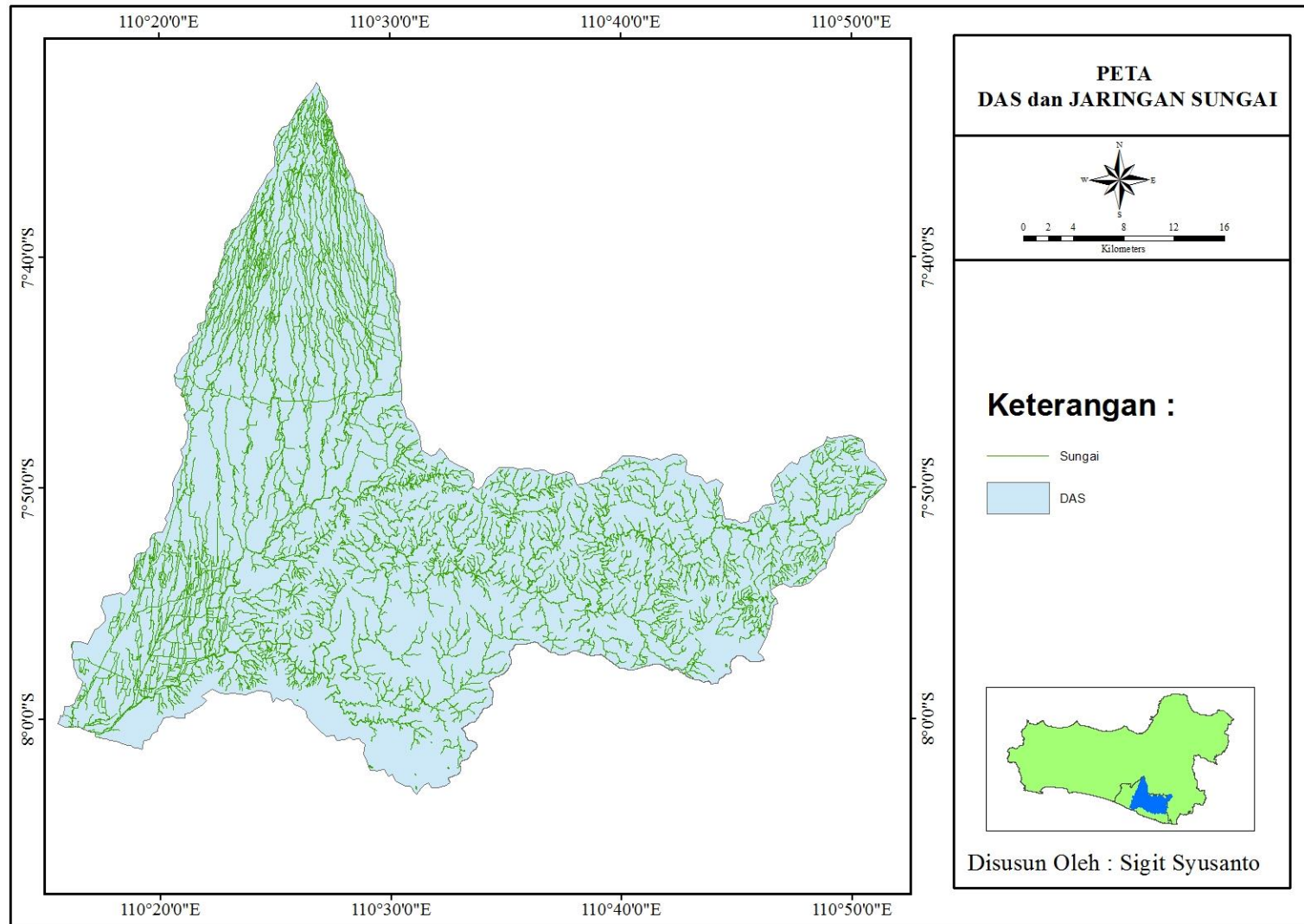
Gambar 6. Peta Jaringan dan Batas DAS Sungai Opak-Oyo Dari Balai Pengelolaan Daerah Aliran Sungai (BPDAS)
